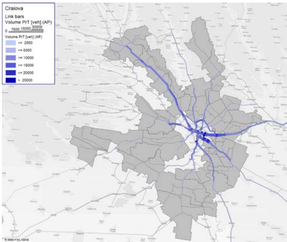
Figură 3-39 Fluxuri de vehicule afectate pe rețeaua de referință – nivel metropolitan, anul 2021
