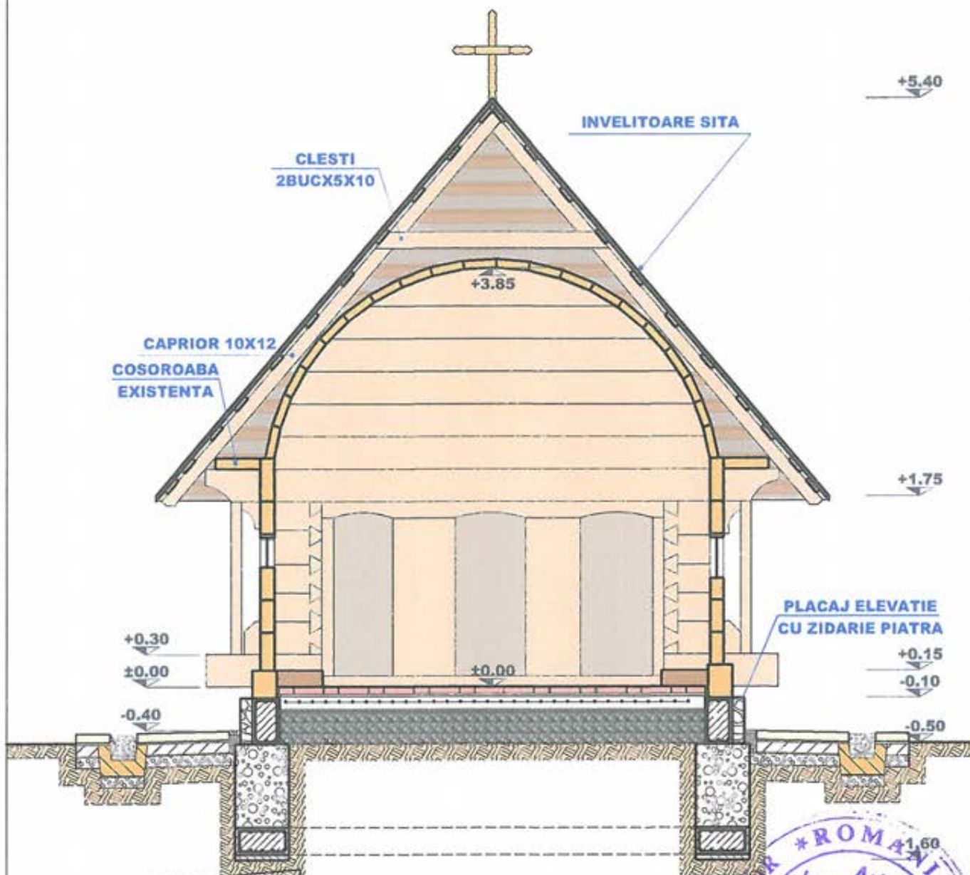
SECTIUNEA b-b scara 1:50
