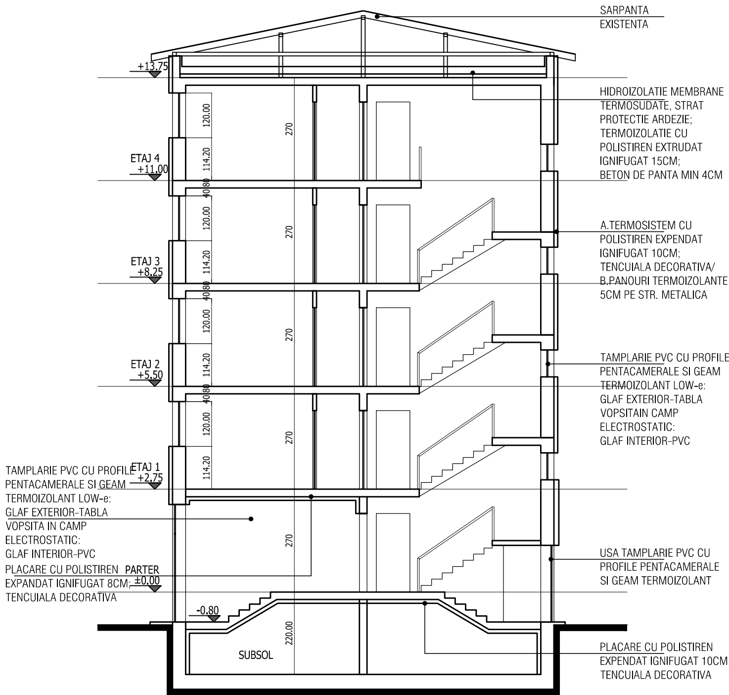
SECTIUNE TRANSVERSALA - PROPUNERE
