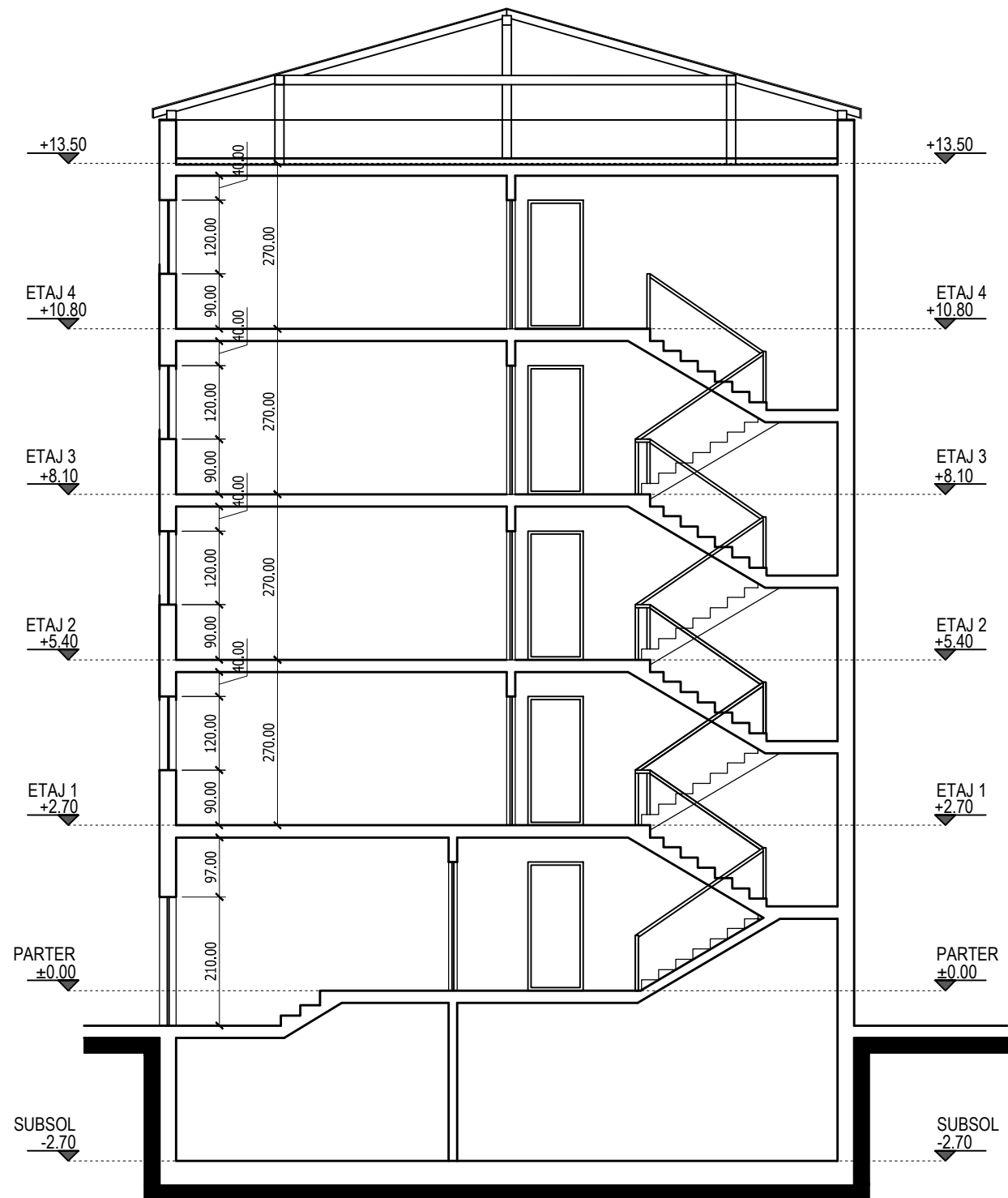
SECTIUNE TRANSVERSALA - RELEVU
