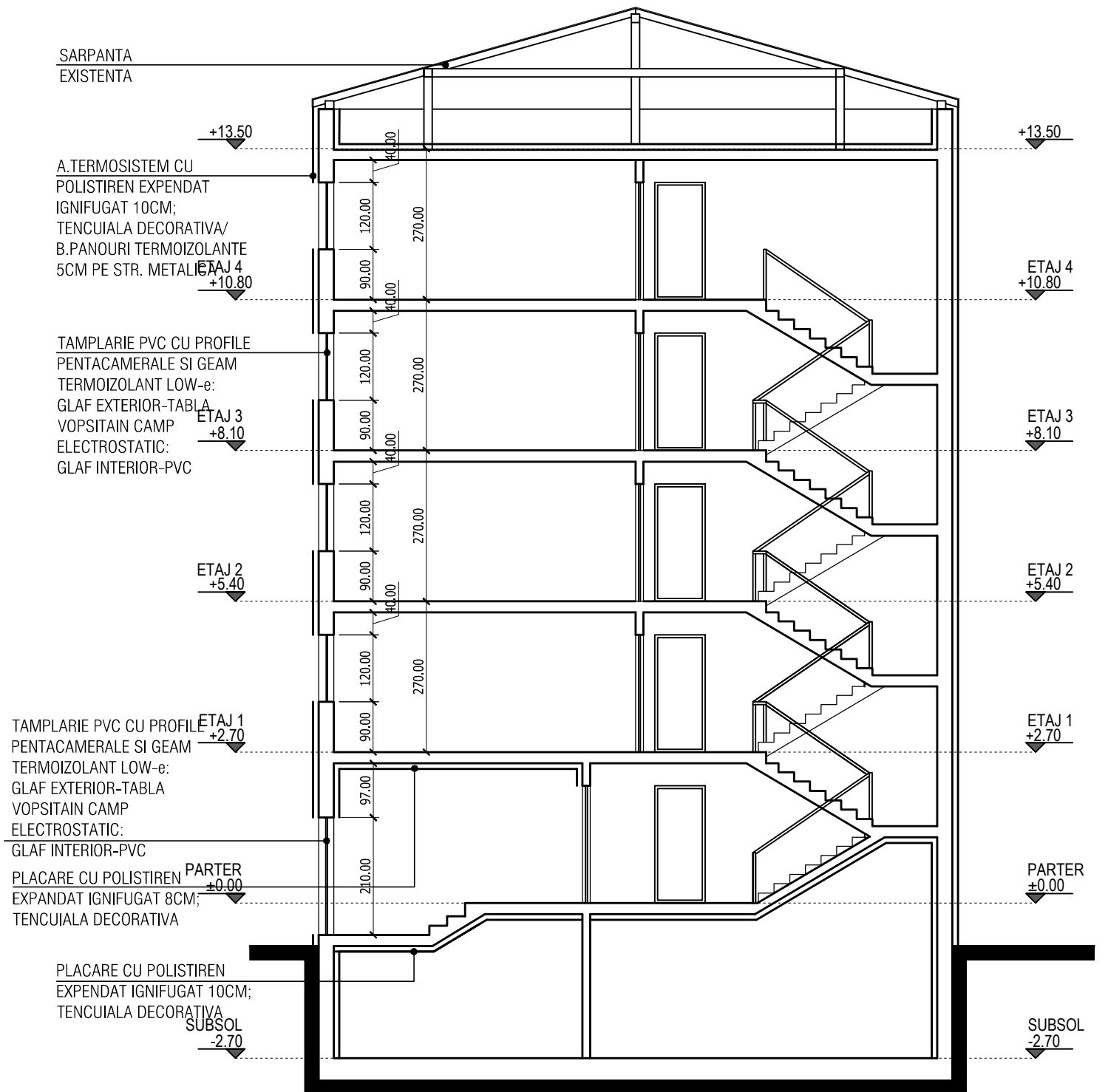
SECTIUNE TRANSVERSALA - PROPUNERE
