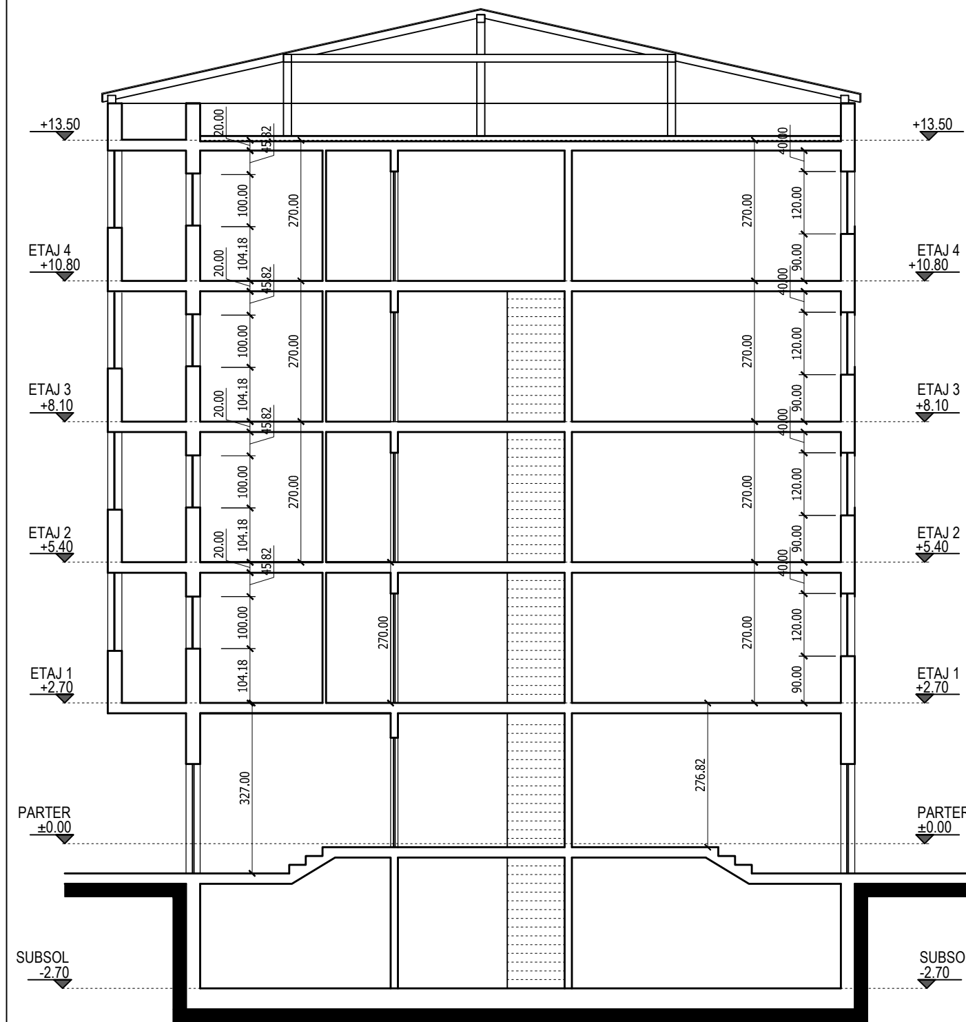
SECTIUNE TRANSVERSALA - RELEVU
