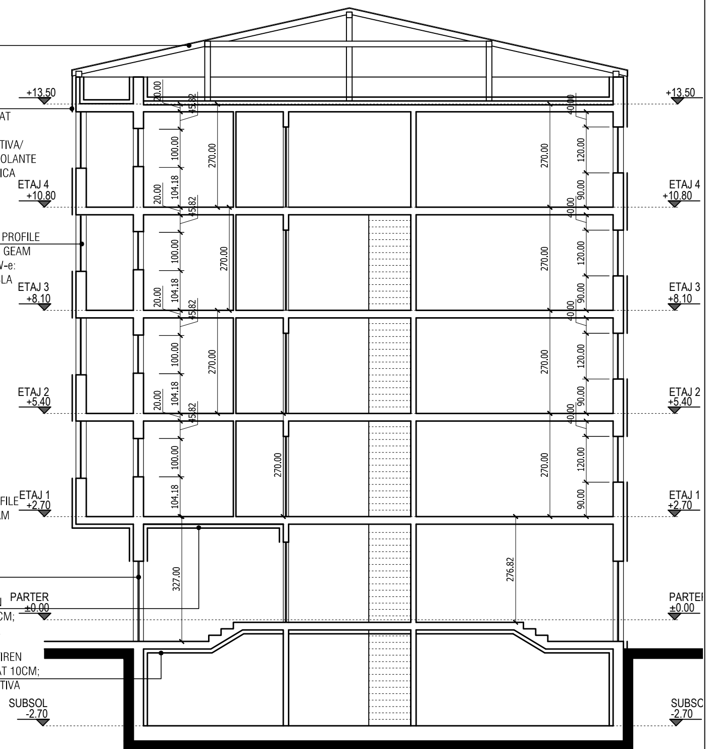
SECTIUNE TRANSVERSALA - PROPUNERE
