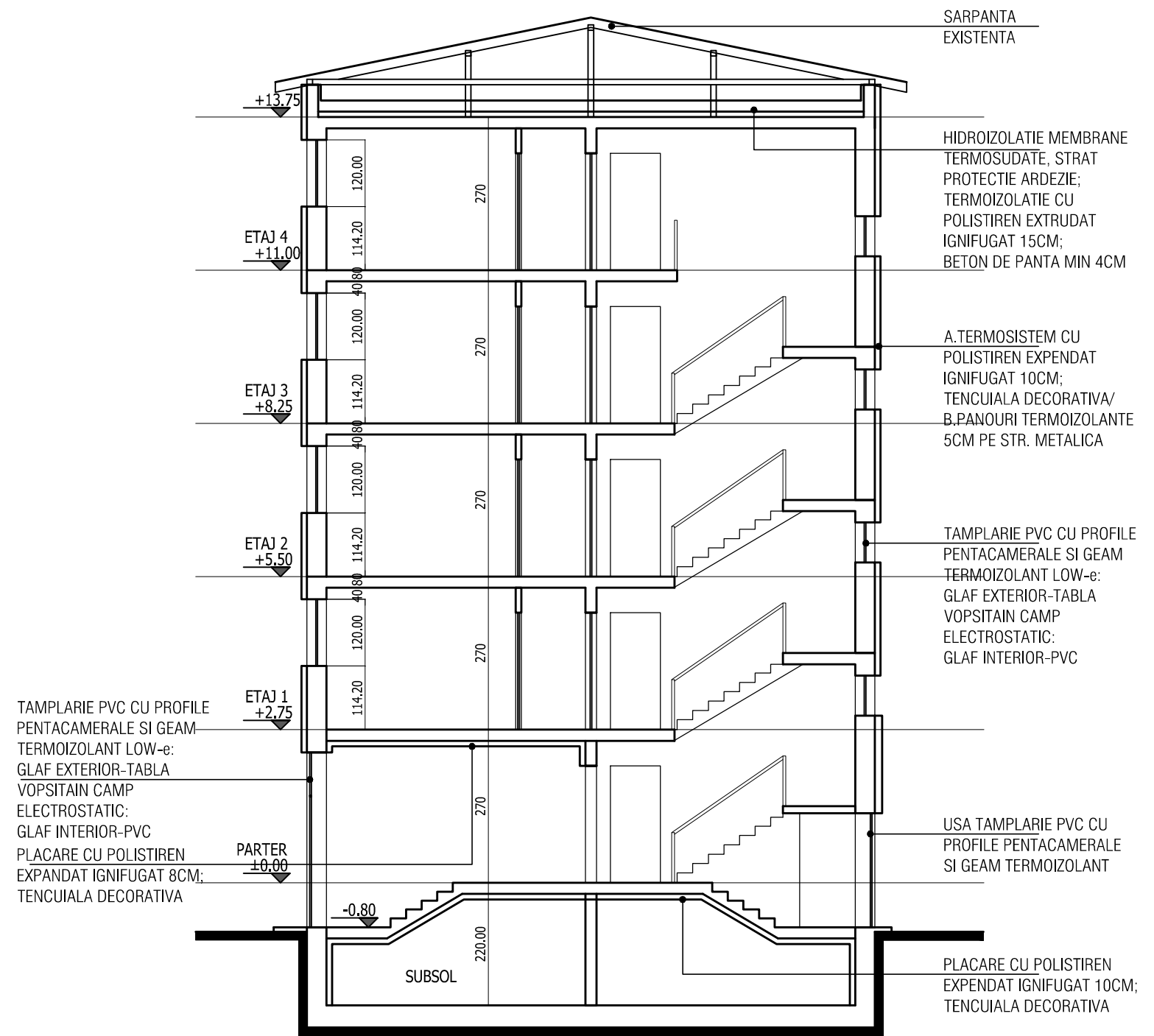
SECTIUNE TRANSVERSALA - PROPUNERE
