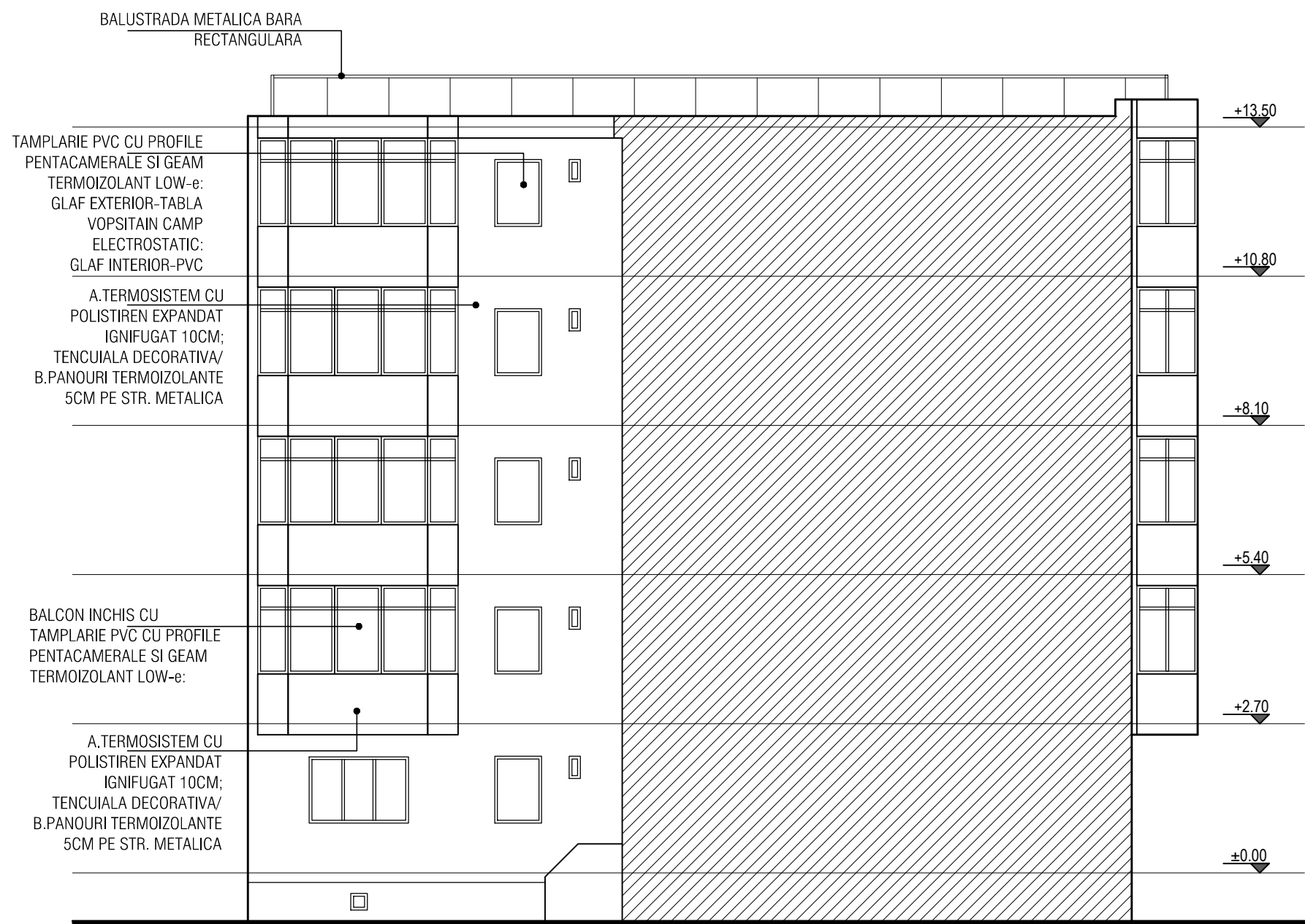
FATADA POSTERIOARA FATADA POSTERIOARA
