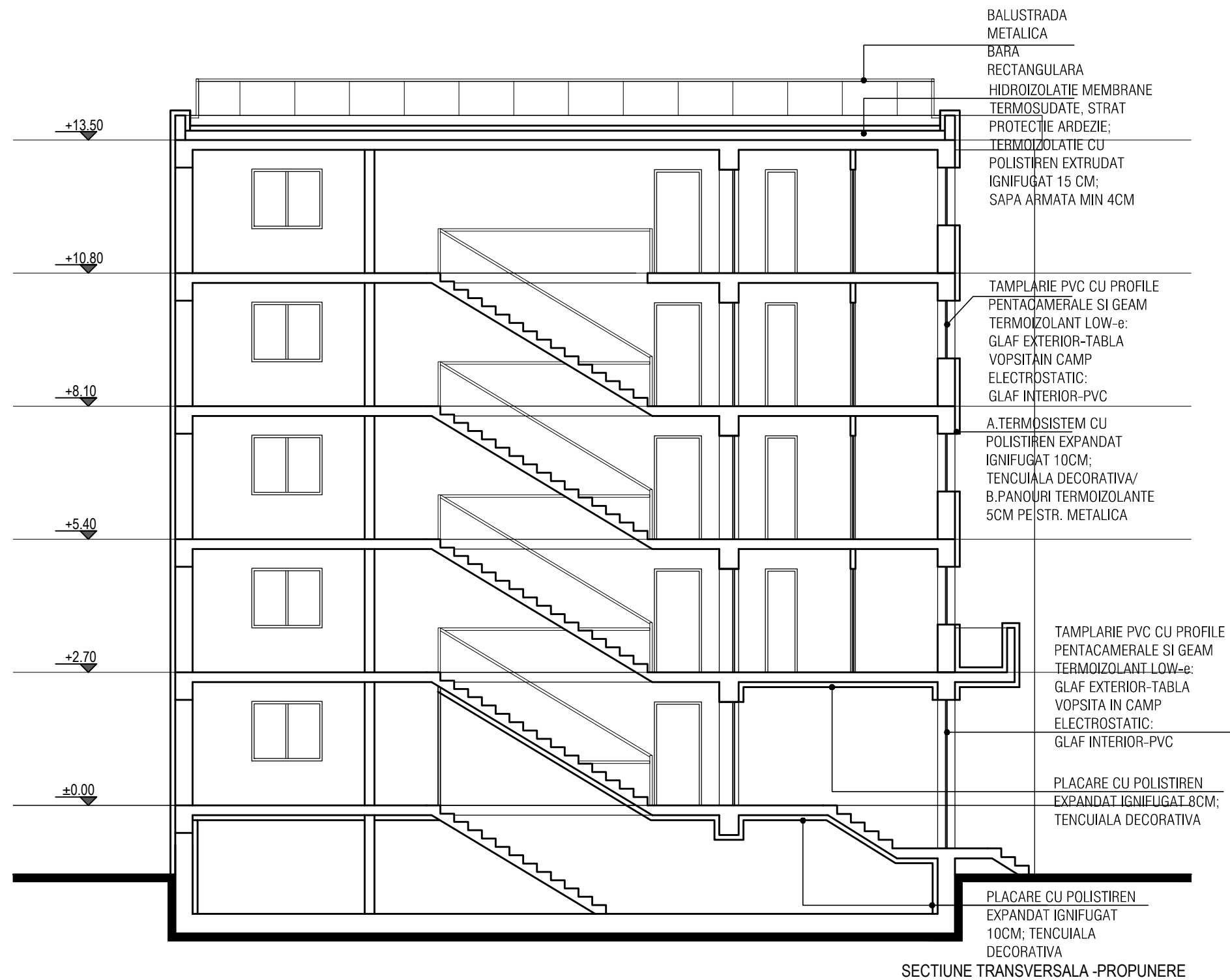
SECTIUNE TRANSVERSALA -PROPUNERE
