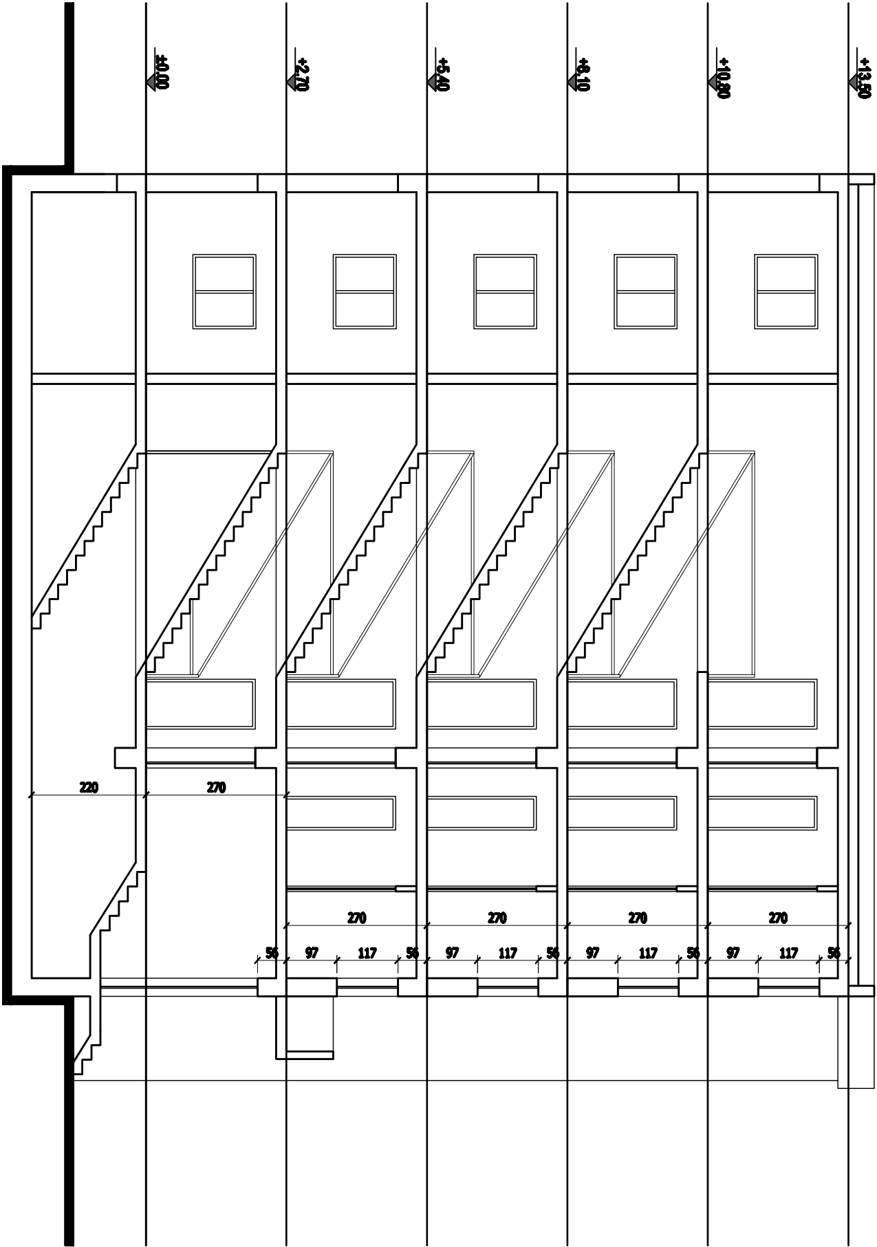
SECȚIUNE TRANSVERSALA -PROFUNDIERE
