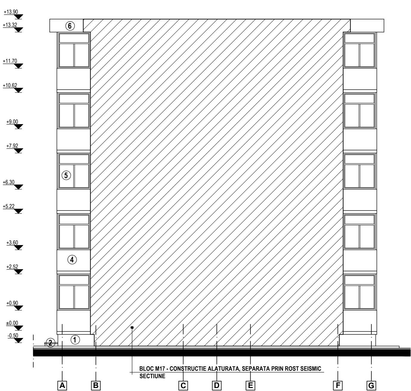
FATADA LATERALA DREAPTA
