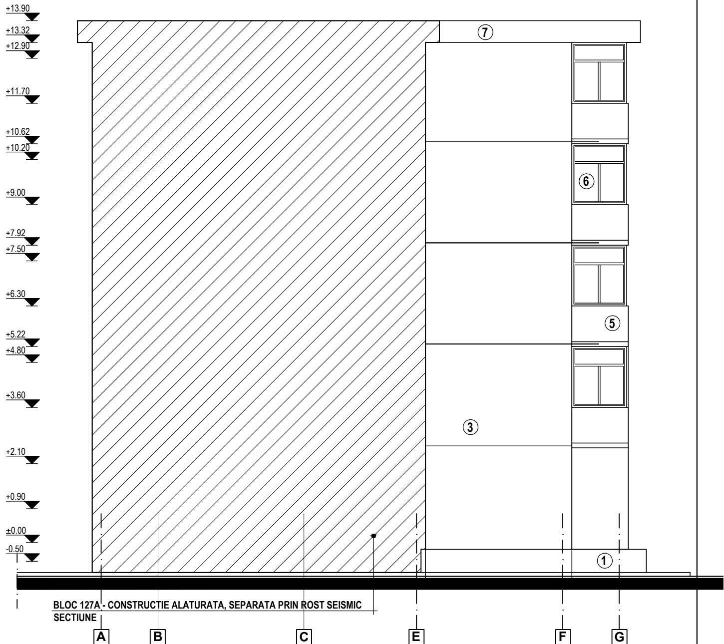
FATADA LATERALA DREAPTA
