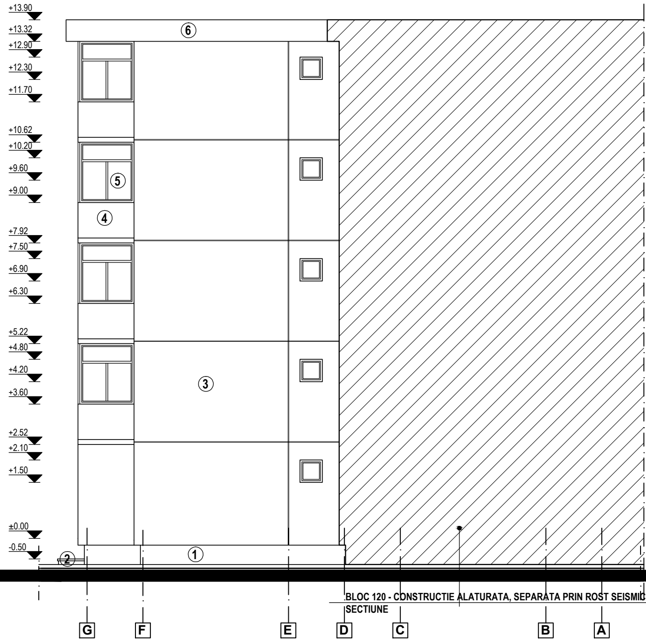
FATADA LATERALA DREAPTA
