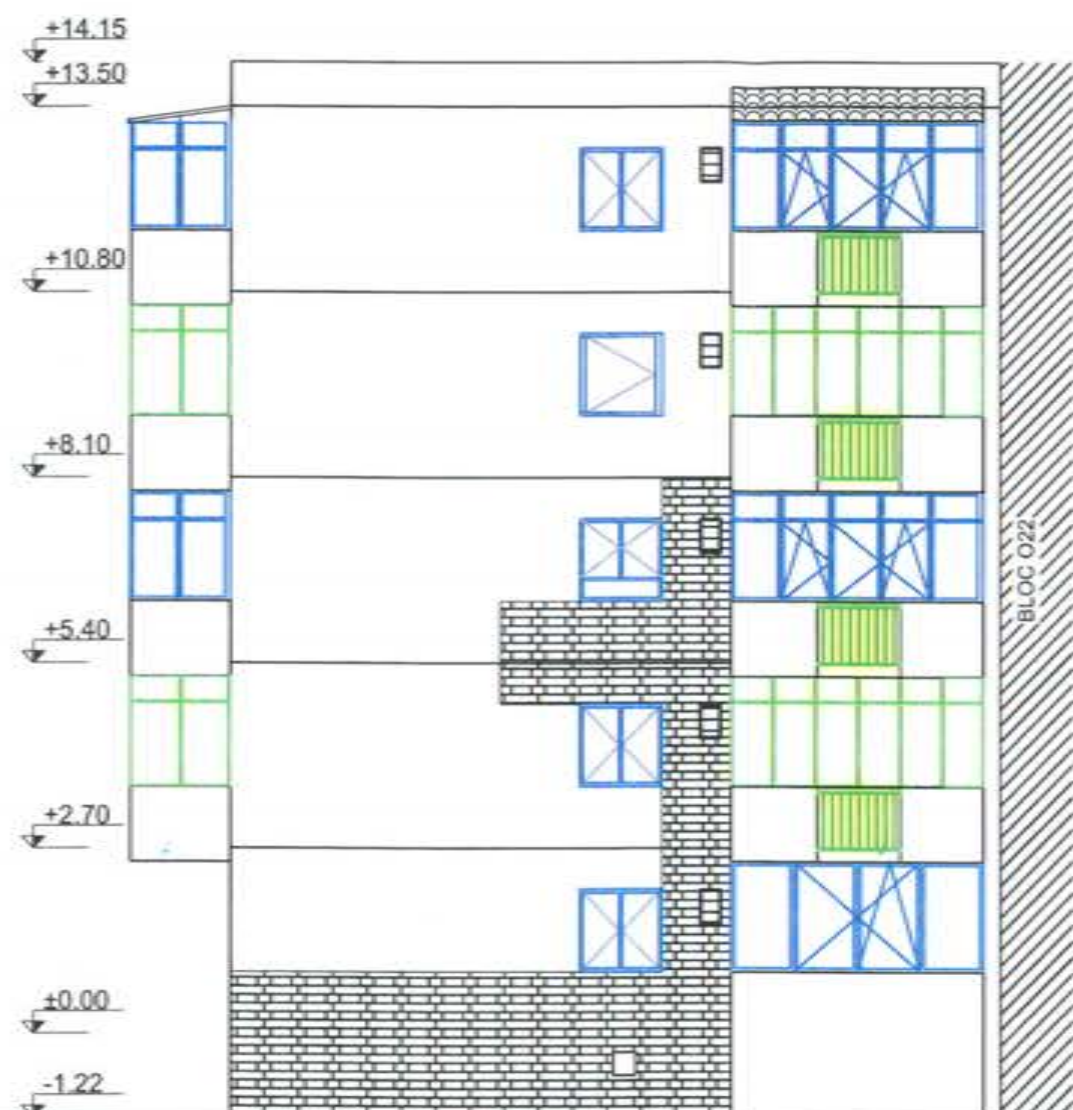
O21 Scara 2 FATADA LATERALA DREAPTA (VEST)
