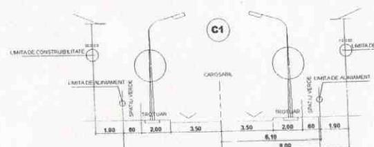
C/C1 STRAZI DE CATEGORIA A III-a - colectoare - cu 2 benzi
