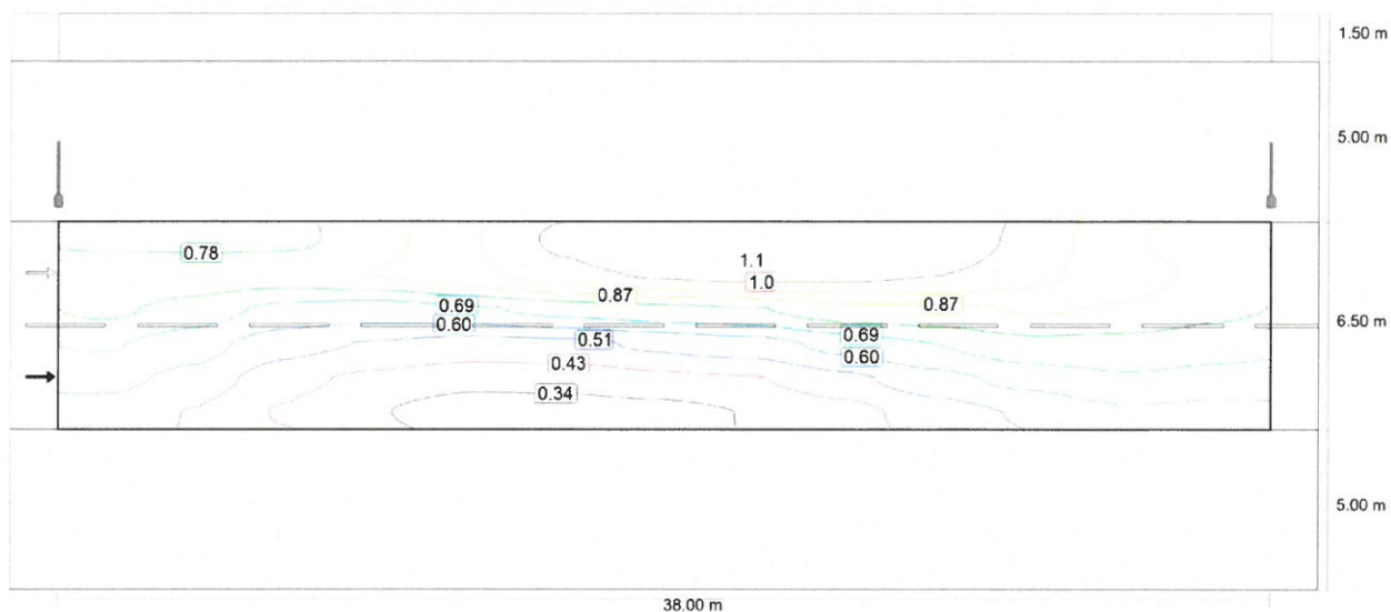
Observator 1: Valoarea de întreținere, densitatea luminii cu carosabil uscat [ \text{cd/m}^2 ] (Linii Isolux)
