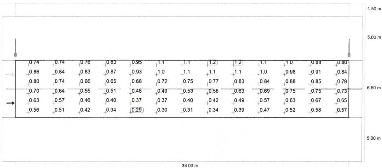
Observator 1: Valoarea de întreținere, densitatea luminii cu carosabil uscat [ \text{cd/m}^2 ] (Raster valoric)
