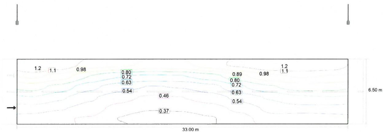
Observator 1: Densitatea luminii la instalația nouă [cd/m²] (Linii Isolux)
