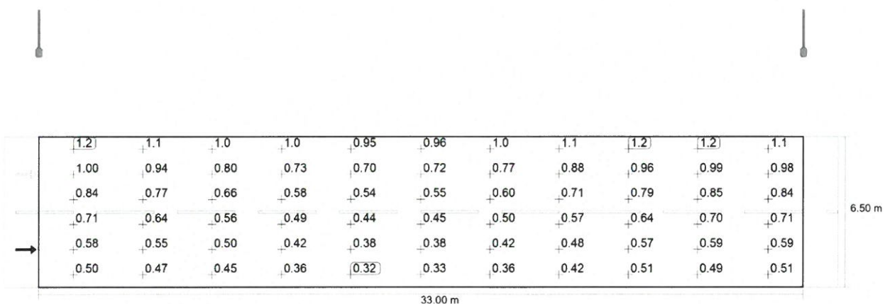
Observator 1: Densitatea luminii la instalația nouă [cd/m²] (Raster valoric)
