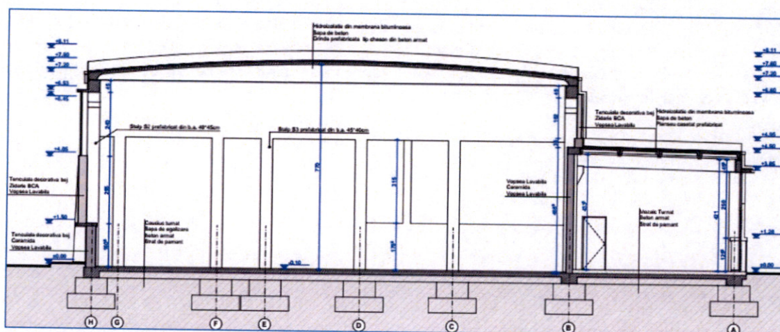
Secțiune transversală existentă
