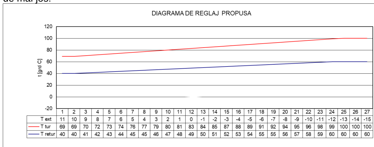
Figura 33. Diagrama de reglaj temperatura termoficare propusă
