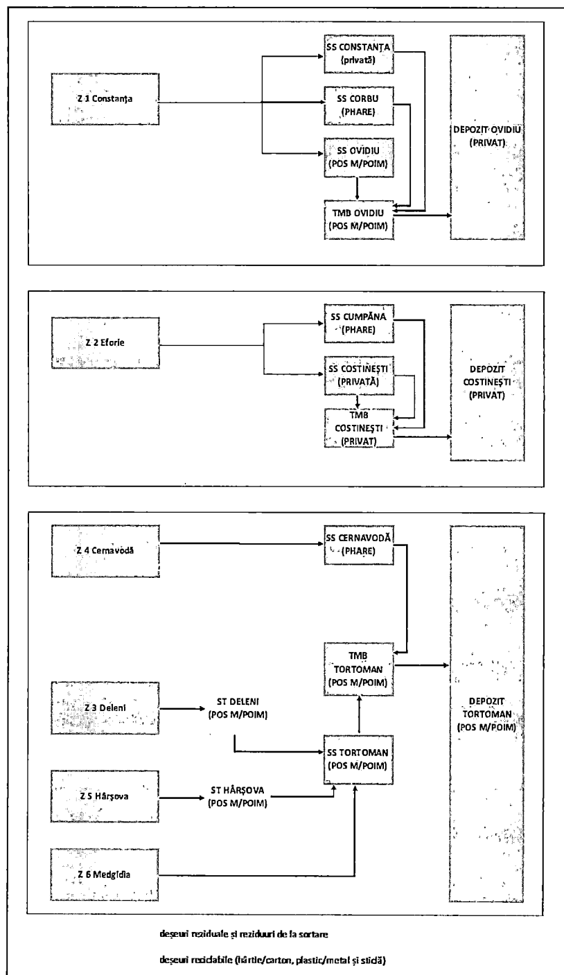
Figura 9-2: Sortarea deșeurilor reciclabile colectate separat
