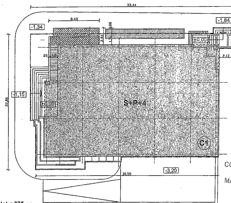
PLAN DE SITUATIE SC: 1:250
