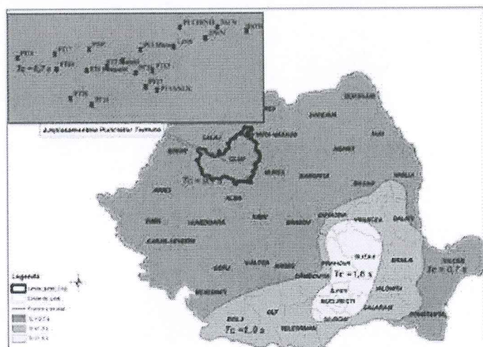
Figură 5-4: Harta zonării seismice în termeni de perioada de control (colț) T_c a spectrului de răspuns
