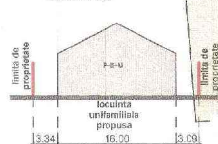
PROFIL LONGITUDINAL 2-2 SCARA 1:500
