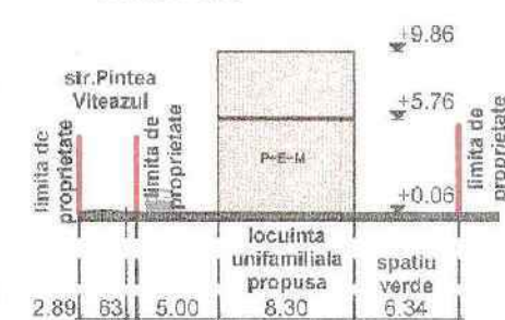
PROFIL TRANSVERSAL 1-1 SCARA 1:500
