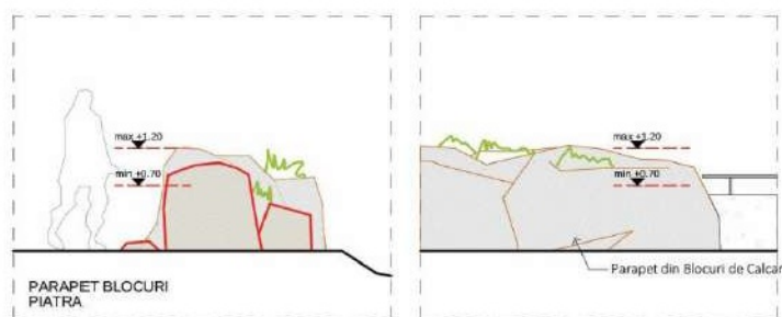
Figura 20 – Parapeți realizați din blocuri de piatră cu fundații de beton
