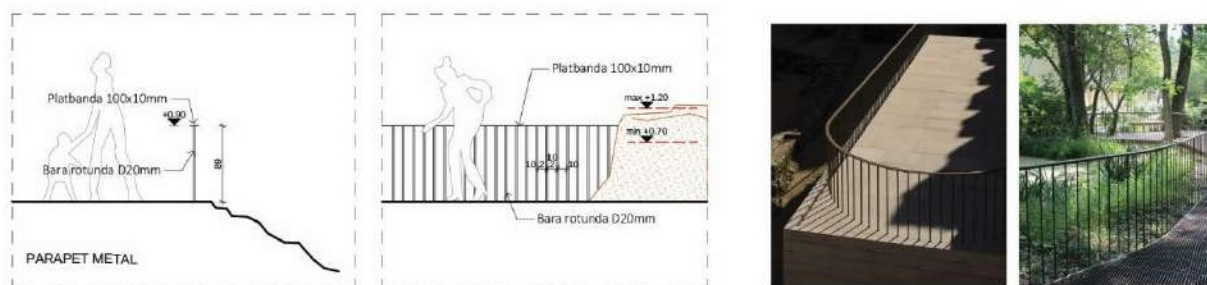
Figura 19 – Parapeți metalici realizați din elemente verticale cu înălțime de 90cm
