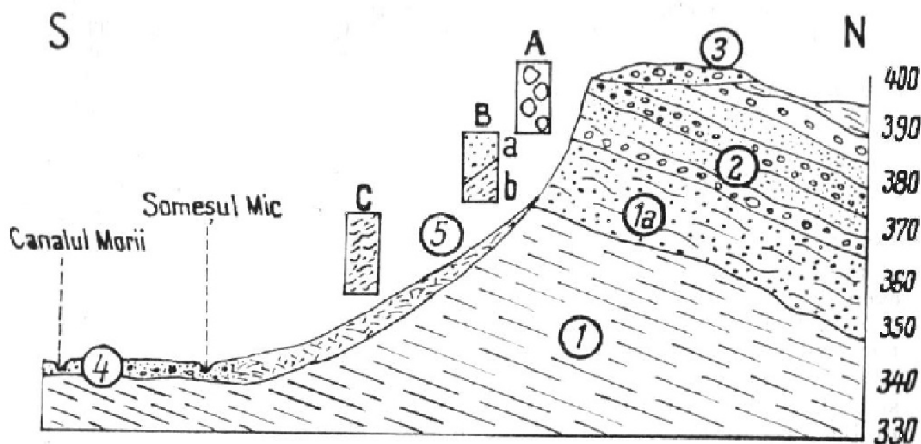
Figura 7 – Profil geologic schematic al dealului Cetățuia (Tövissi, 1989)
