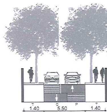
PROFIL STR. E. LOVINESCU ZONA LOCUINTE INDIVIDUALE
