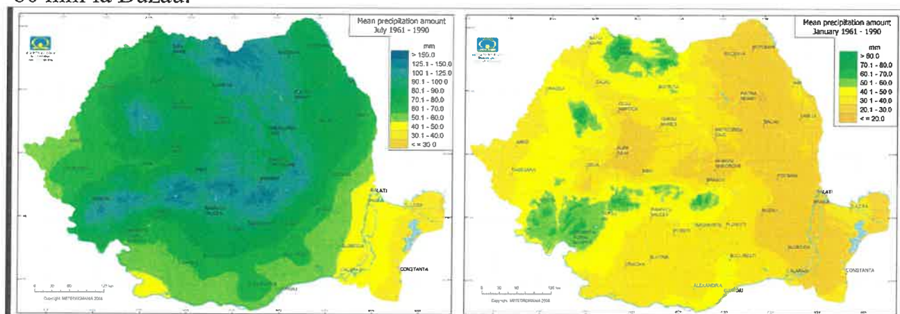
Figura 03. Harta repartiției precipitațiilor medii anuale a României
