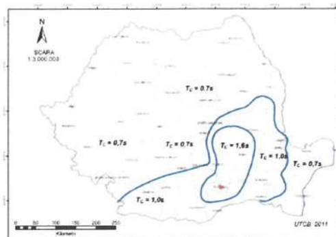
Figura A2 Zona seismică România în termeni de perioada de colț T_c a spectrului de răspuns
