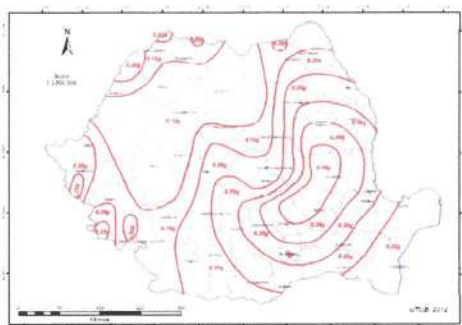
Figura A1 România - Zona de valori de vârf de accelerații seismice pentru proiectare cu IMR = 225 ani și 20% probabilitate de depășire în 50 de ani
