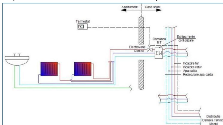
Figura 8. Schema simplificata sistem de incalzire cu distribuție pe orizontală
