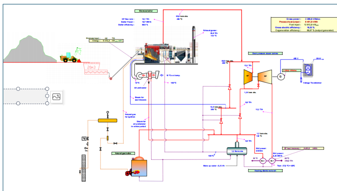
Figura 19. Schema unei centrale de cogenerare pe biomasa
