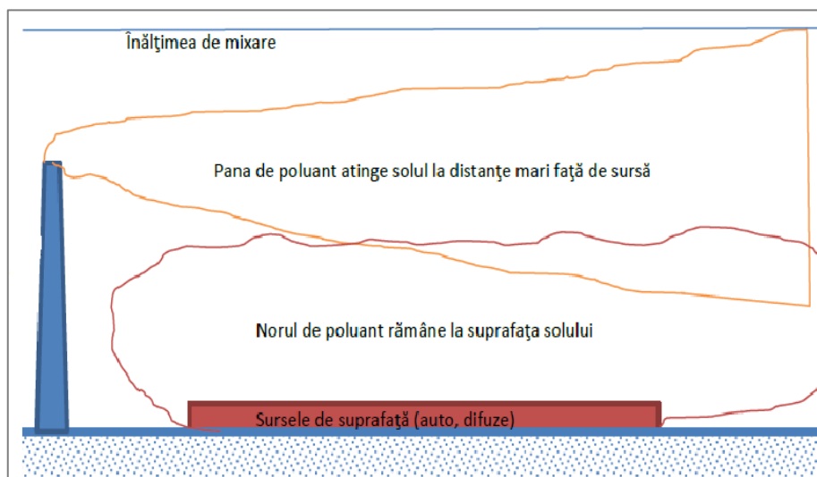
Figura 14. Dispersia emisiilor
