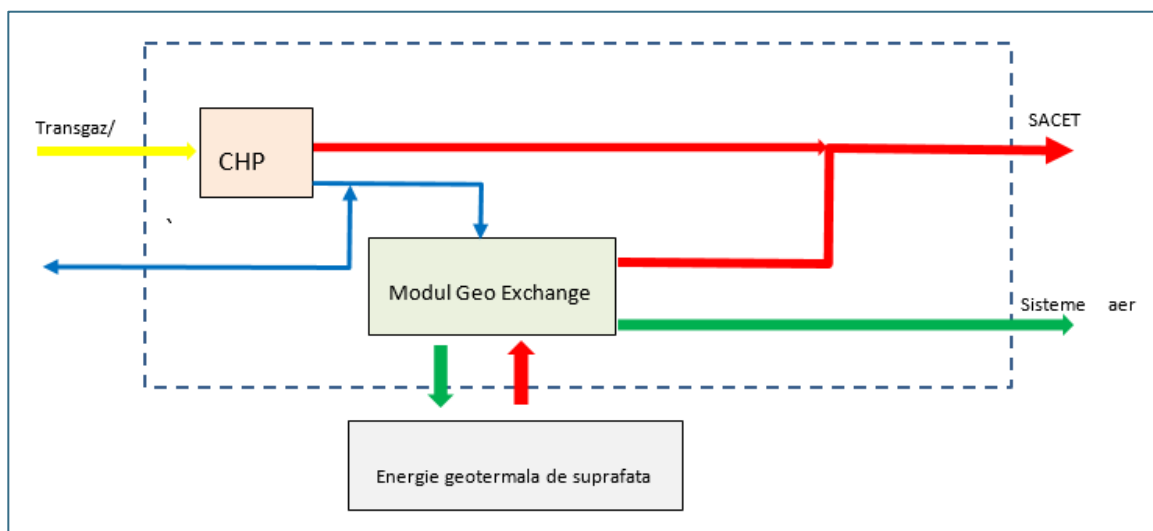
Figura 23. Schema simplificată a unei centrale de cvartal Geo DH/C
