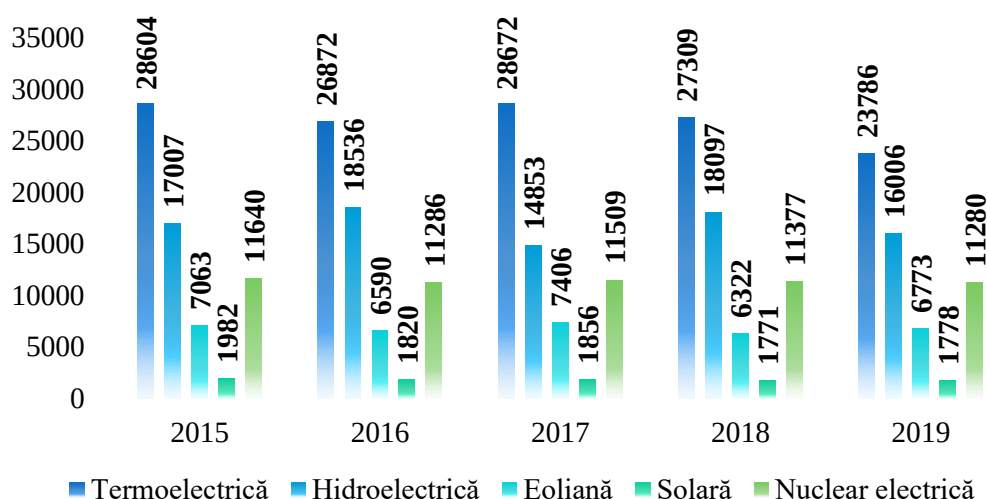
Figura nr. 9 – Producția de energie electrică pe categorii de centrale electrice
