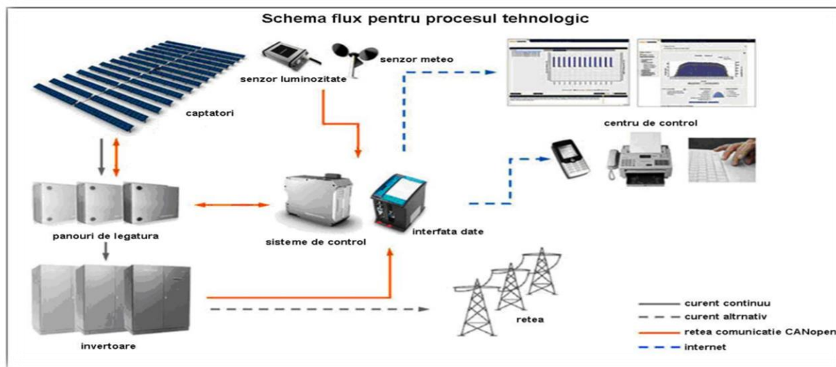
Figura nr. 37 – Schema de funcționare a unui parc fotovoltaic
