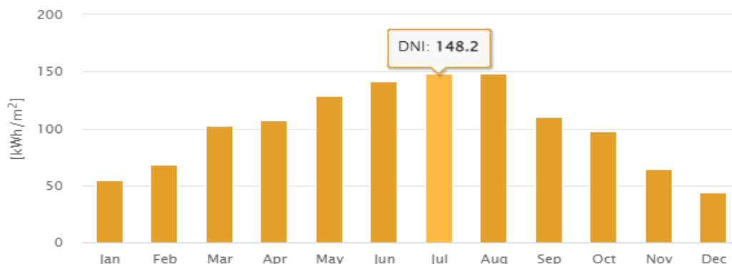
Figura nr. 34 – Iradierea normală directă kWh/ m 2
