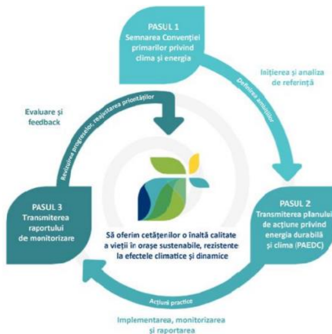
Figura nr. 5 – Procesul Convenției primarilor privind clima și energia pas cu pas
