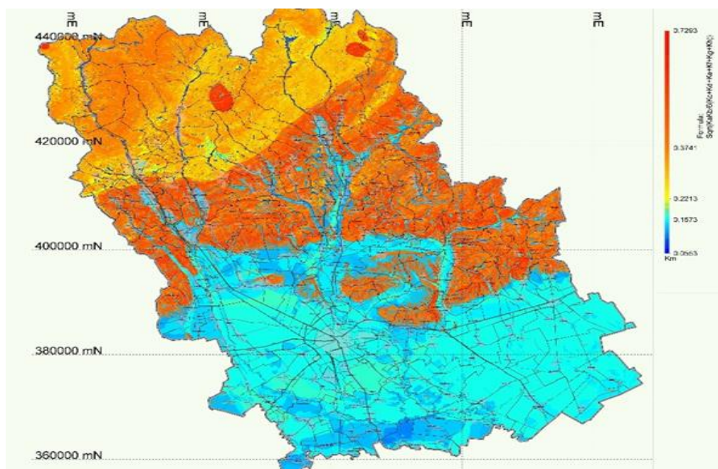
Figura nr. 17 – Mișcarea plăcilor tectonice 24
