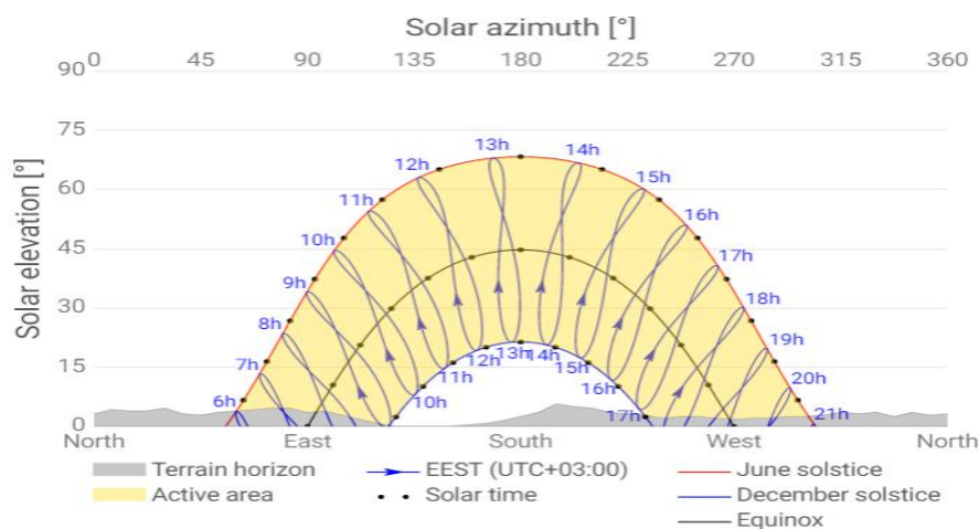
Figura nr. 36 – Azimutul solar – orașul Breaza
