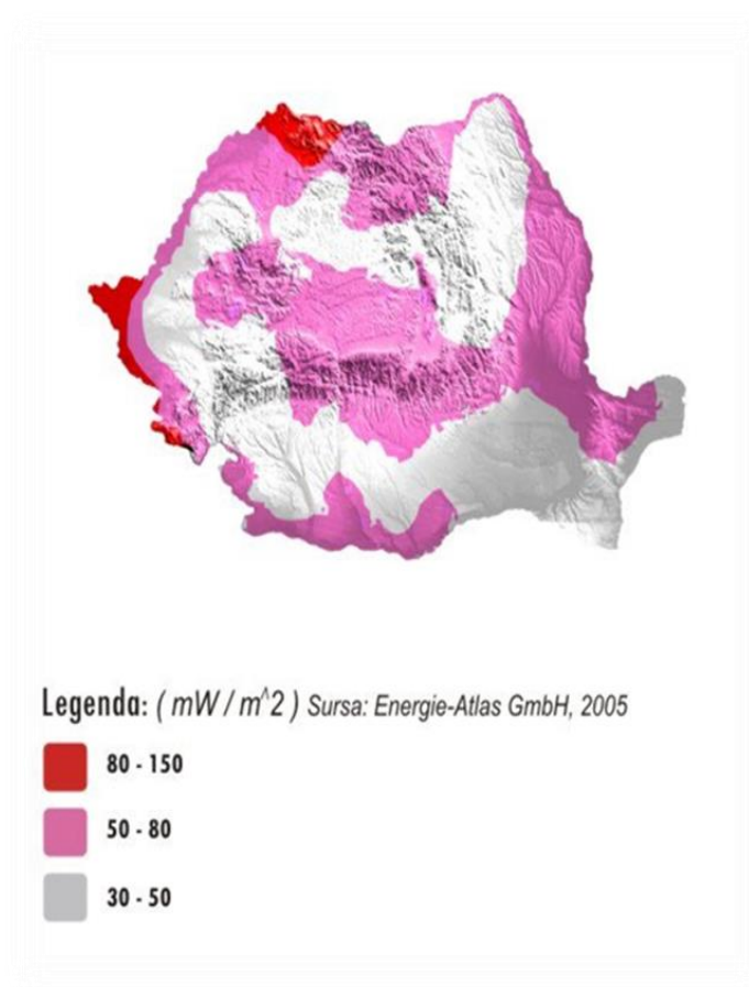
Imagine nr. 13 – Harta cu potențial geotermal al României
