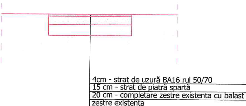
Detaliu de executie S3 scara 1:40
