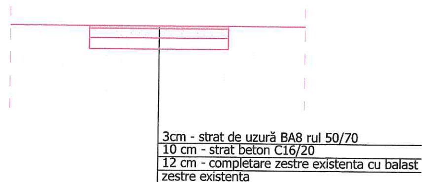
Detaliu de executie ST2 scara 1:40
