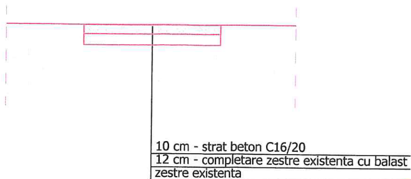
Detaliu de executie ST3 scara 1:40
