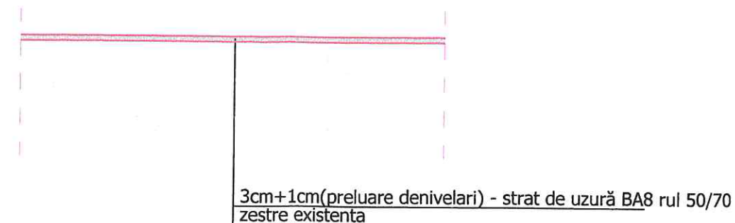
Detaliu de executie ST1 scara 1:40
