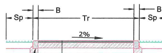
Detaliu de executie S4 -trotuar intrare profesori scara 1:40
