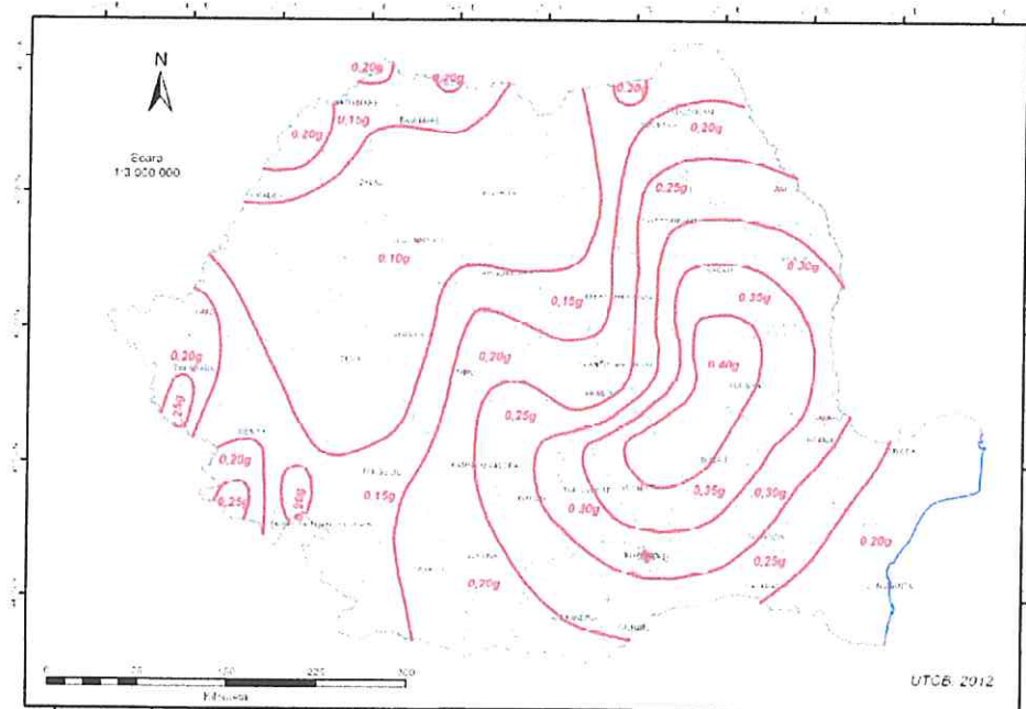
Figura 2 Zonarea valorilor de vârf ale acceleraţiei terenului pentru proiectare
