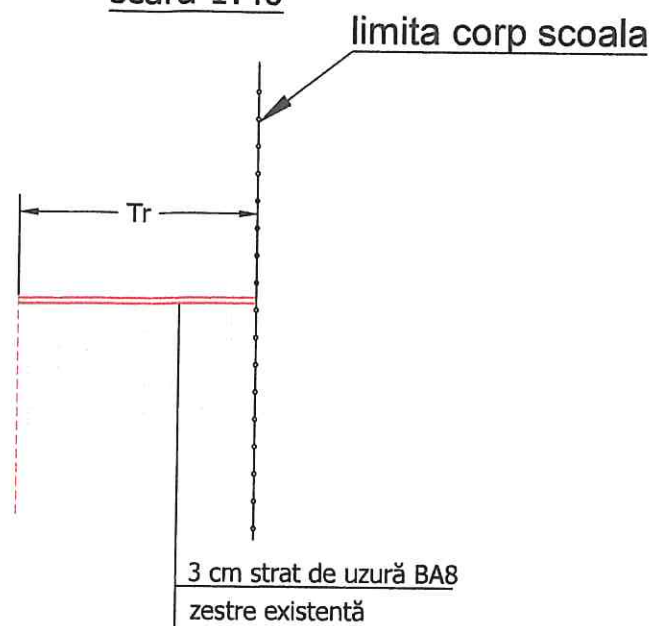
Detaliu de executie S2 scara 1:40
