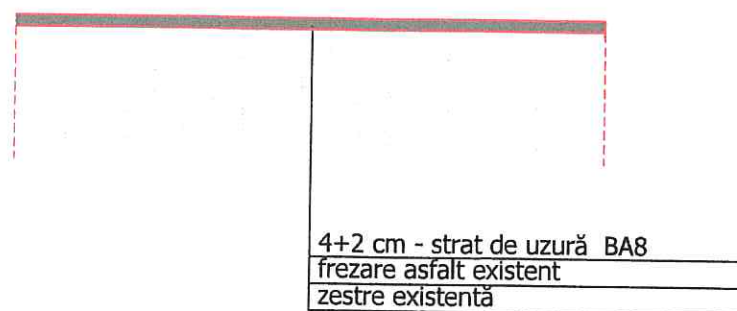
Detaliu de executie S1 scara 1:40
