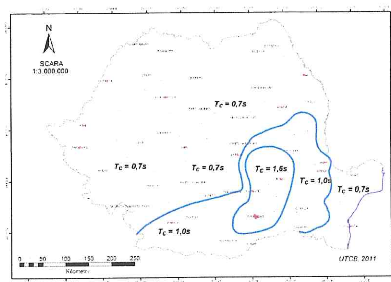
Figura 3 Zonarea teritoriului României în termeni de perioada de control (colț) Date climatice
