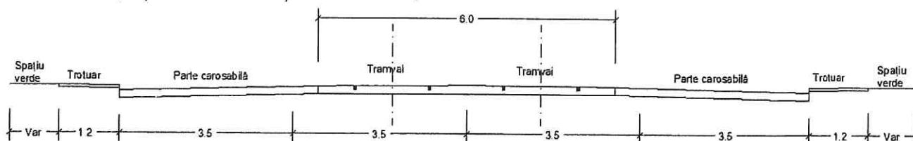
Figura 2: Prospectul tramei stradale Șoseaua Baldovinești și strada Apollo
