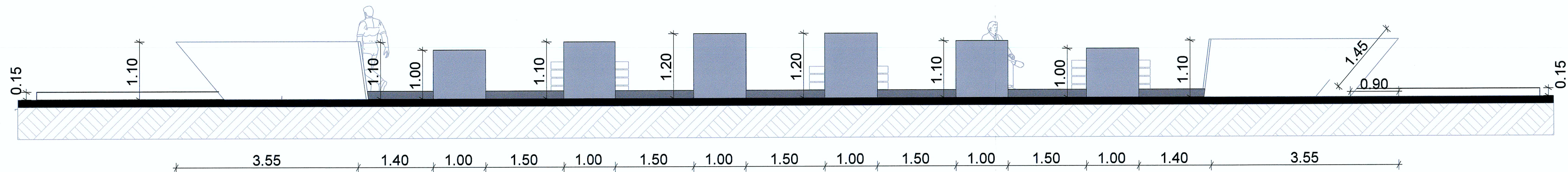
VEDERE LONGITUDINALA
