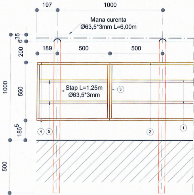
DETALIU A Sc. 1:20
