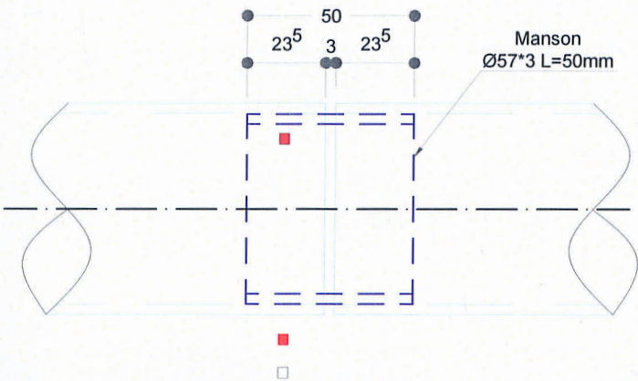
DETALIU C Sc. 1:2
