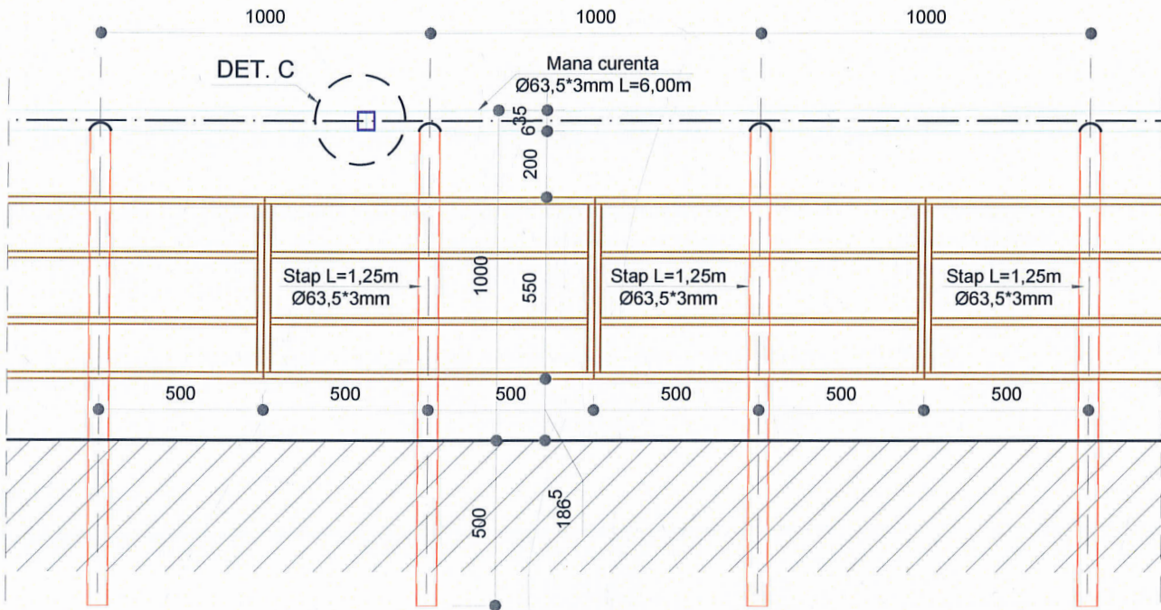
DETALIU B Sc. 1:20
