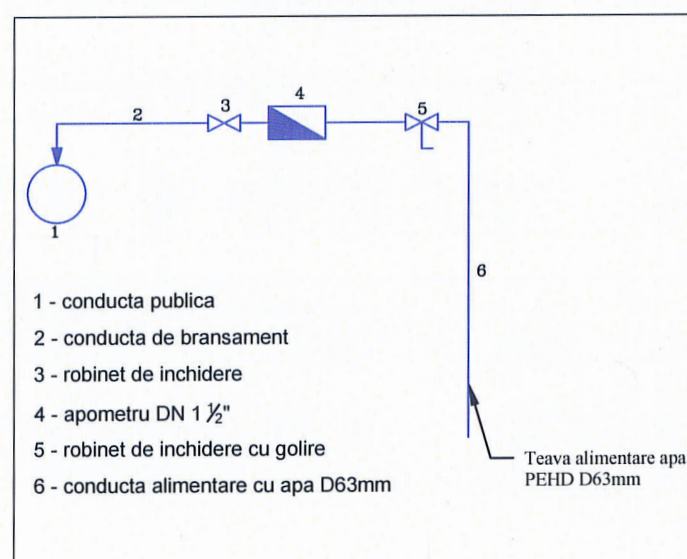
Detaliu camin bransament - CB
