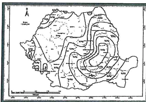
Zonarea valorii de varf a accelerației terenului pentru cutremure având IMR = 225 ani.
