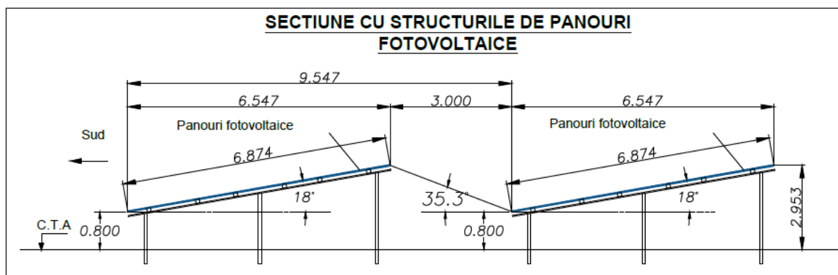
Figura 14. Vedere laterala de principiu a sistemului de montaj montat la sol
