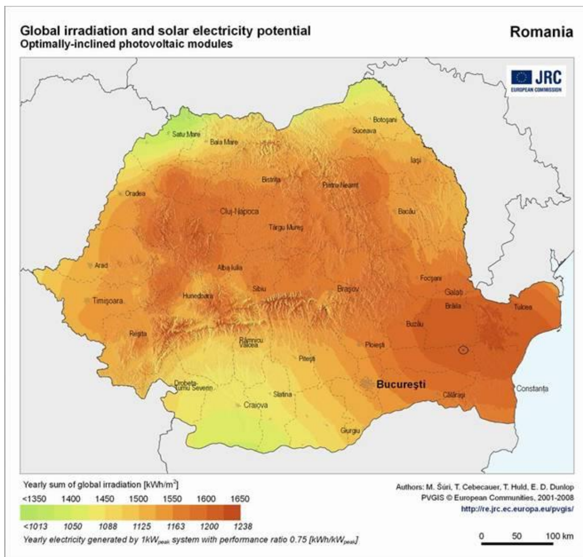
Figura 6. – Potențial Solar Energetic Anual - Panouri Fotovoltaice cu Înclinare 20Gr
