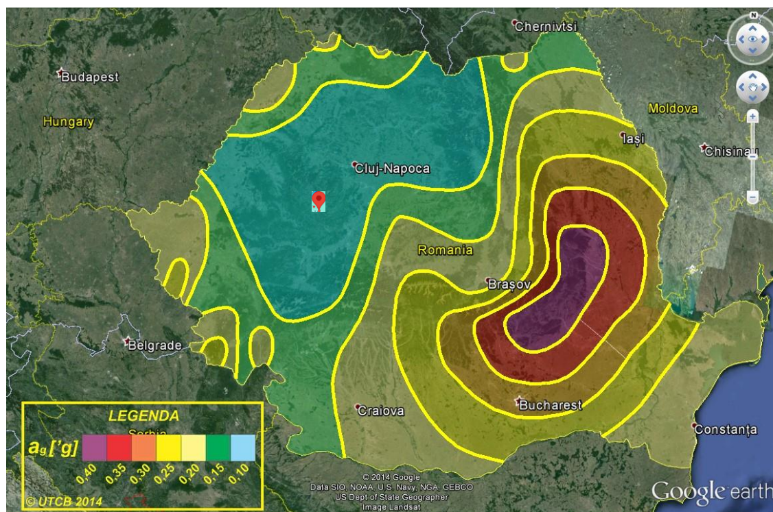
Figura 7. Harta de zonare din codul P100-1/2013
