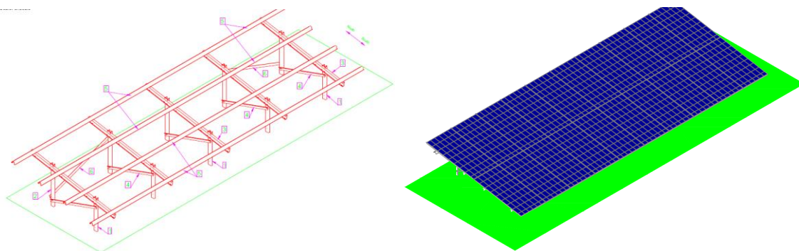
Figura 13. Model de structura metalica de montaj panouri fotovoltaice
