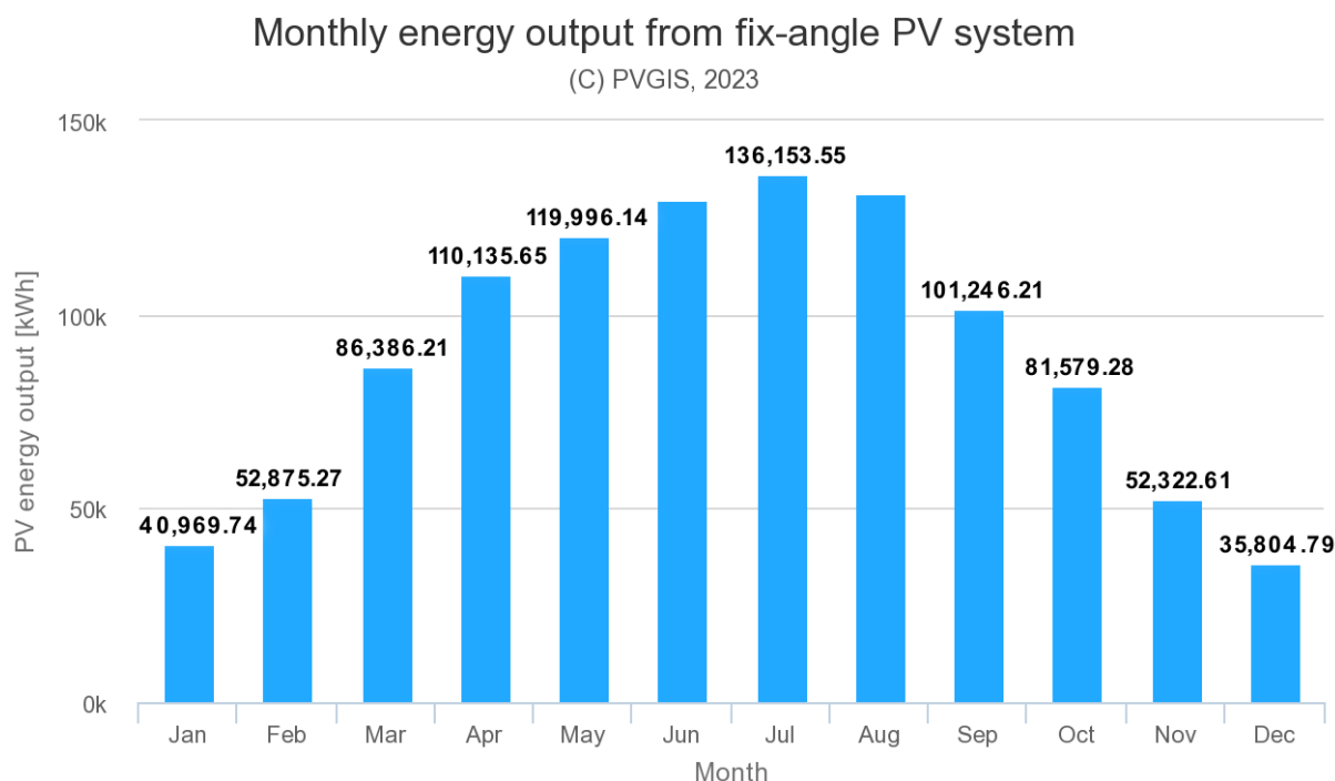
Figura 8. – Producția medie lunară estimată de energie din sursa regenerabilă
