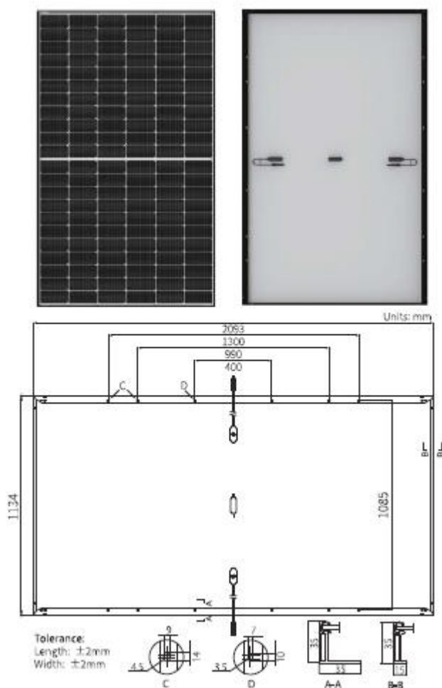
Figura 9. – Model de panou fotovoltaic
