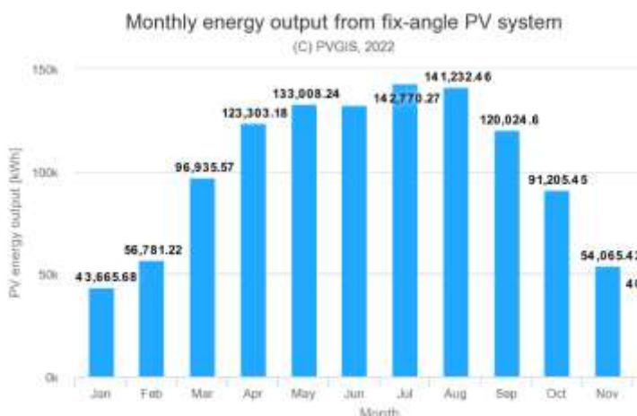
Figura – Cantitatea lunară estimată a energiei electrice de ieșire pentru unghiul fixat
