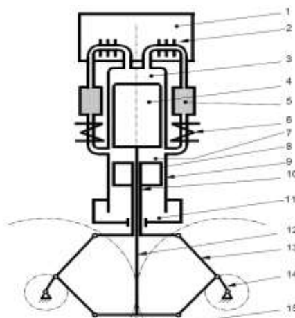
Fig. 1.2. Schema constructivă a motorului Stirling Philips: 1 - cameră de ardere; 2 - încălzitor; 3 - cameră de destindere; 4 - piston împingător; 5 - regenerator; 6 - răcitor; 7 - cameră de comprimare; 8 - piston de lucru; 9 - cilindru; 10 - tija pistonului de lucru; 11 - cameră de amortizare; 12 - tija pistonului împingător; 13 - biela; 14 - arbore cotit; 15 - angrenaj de sincronizare
