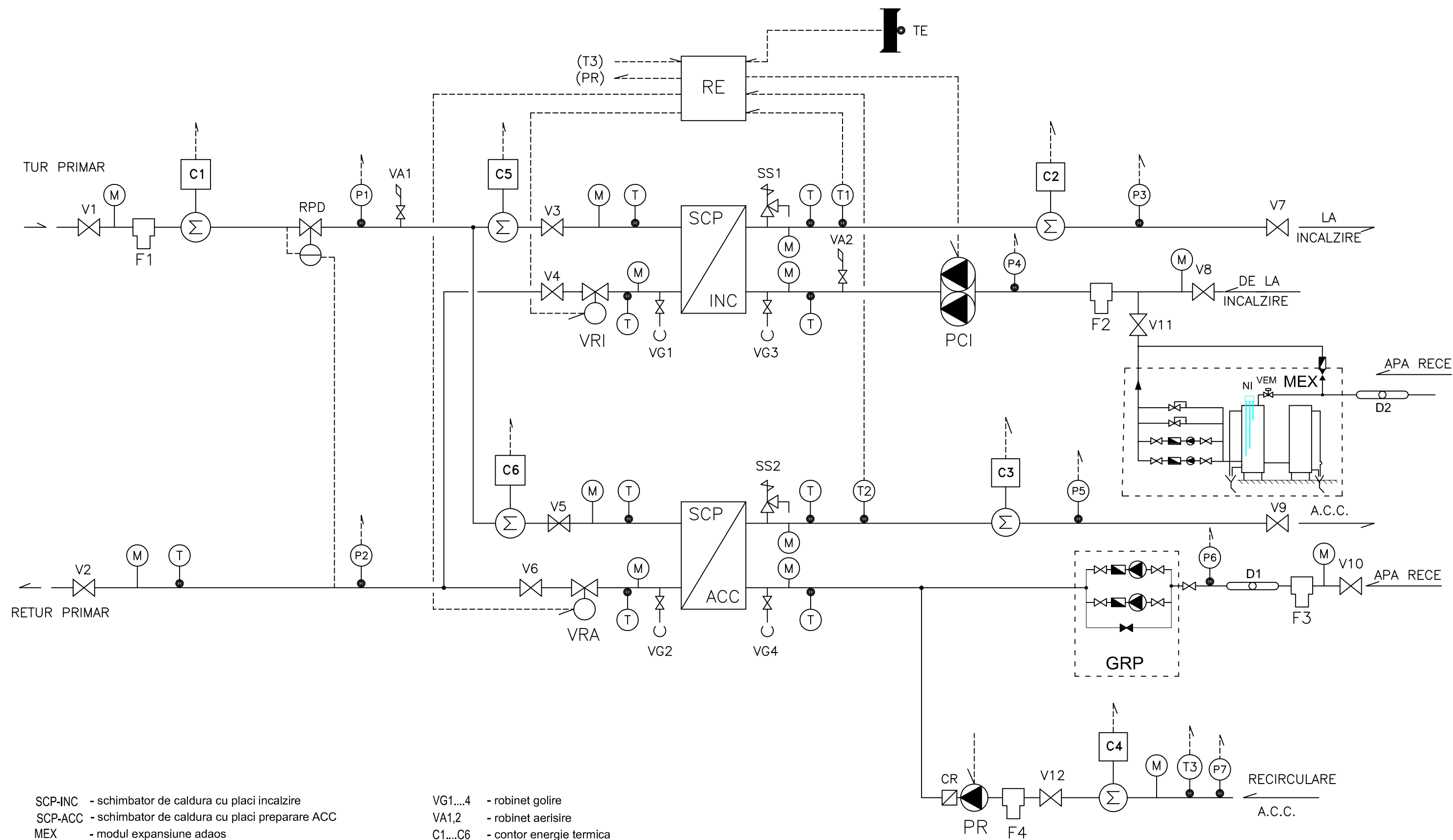
Schema termomecanica Punct Termic centralizat in SACET Botosani cu modul de adaos expansiune in circuitul de incalzire ( in 18 PT)
