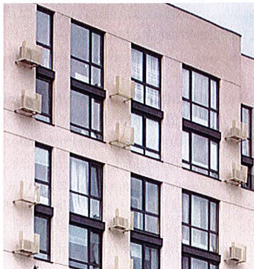
Exemplu de mascare a aparatelor de aer condiționat amplasate pe fațadă cu tablă perforată
