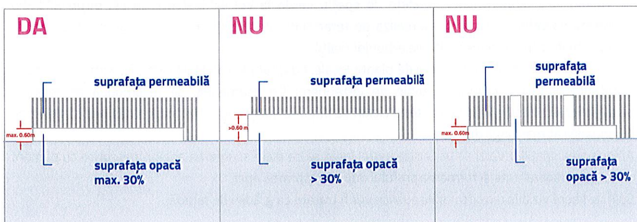
Exemplificarea condițiilor de realizare a împrejmuirilor către aliniament
