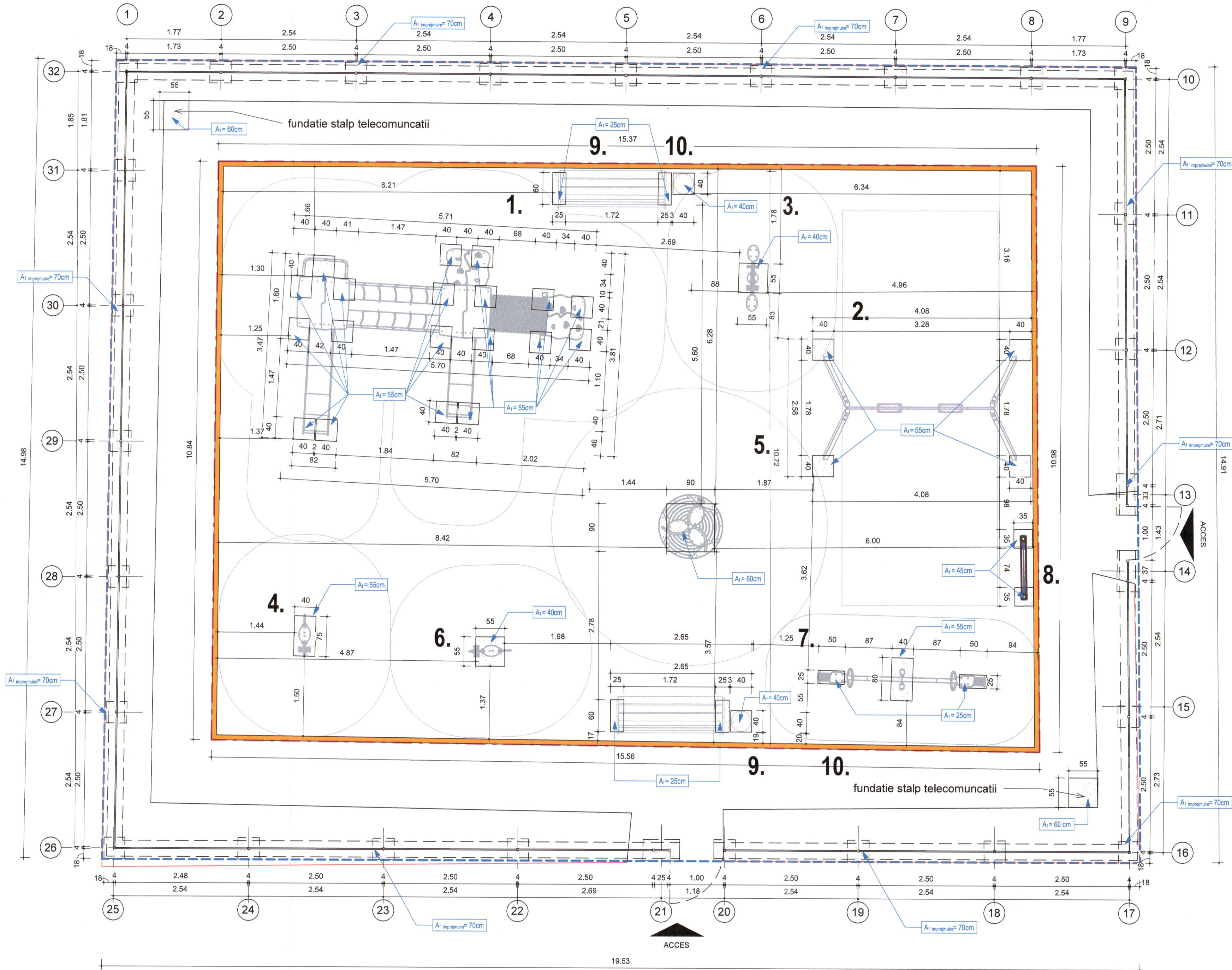
1 Plan fundatii echipamente 1 : 50
