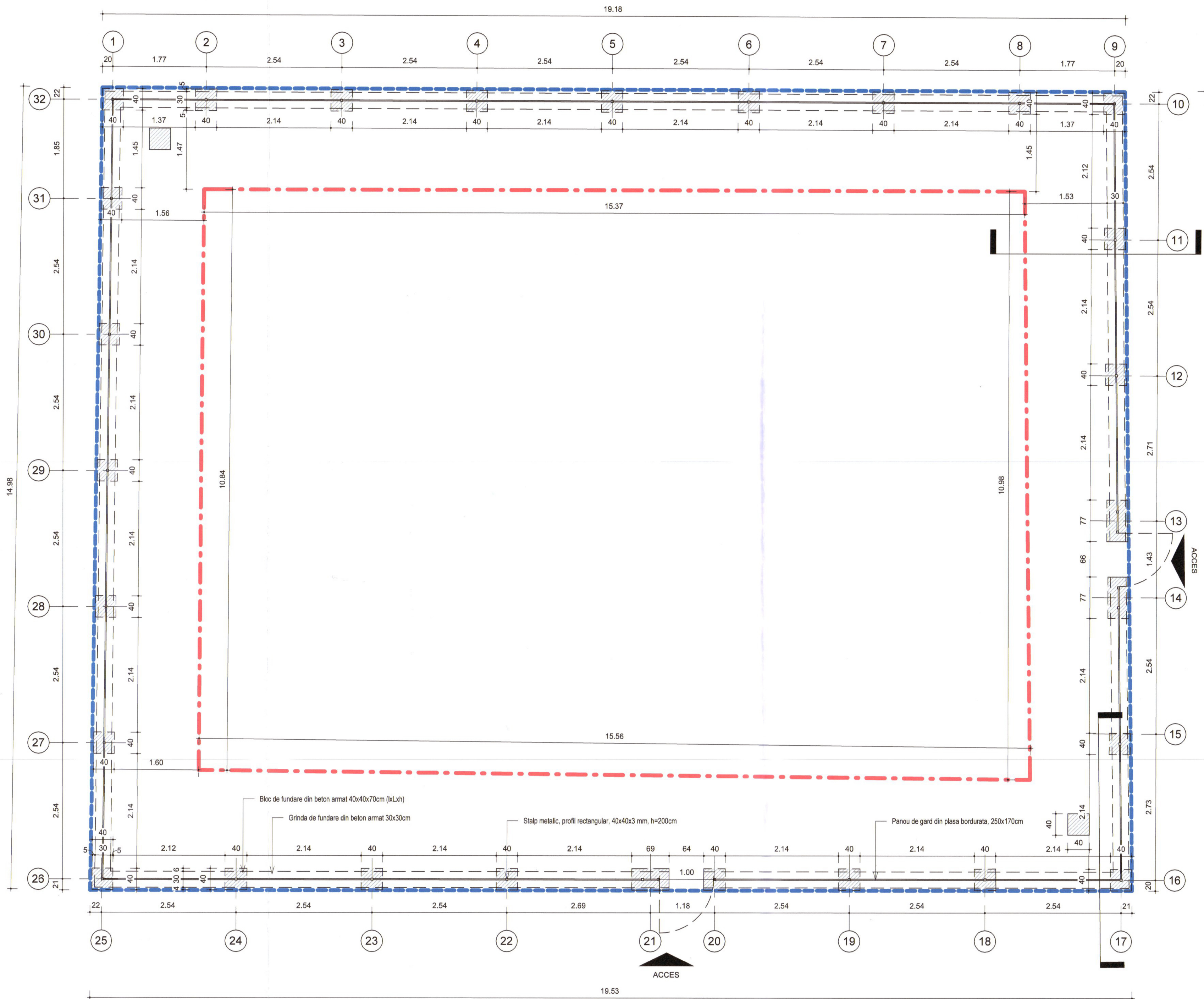
1 Plan fundare imprejmuire 1 : 50
