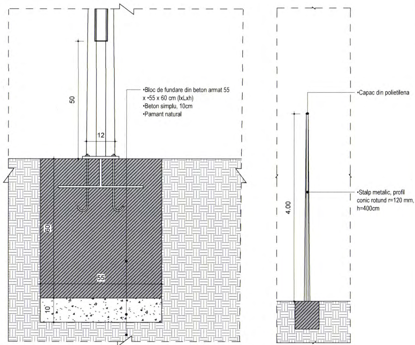
1 Detaliu fundatie si prindere stalp telecomunicatii 1 : 10
