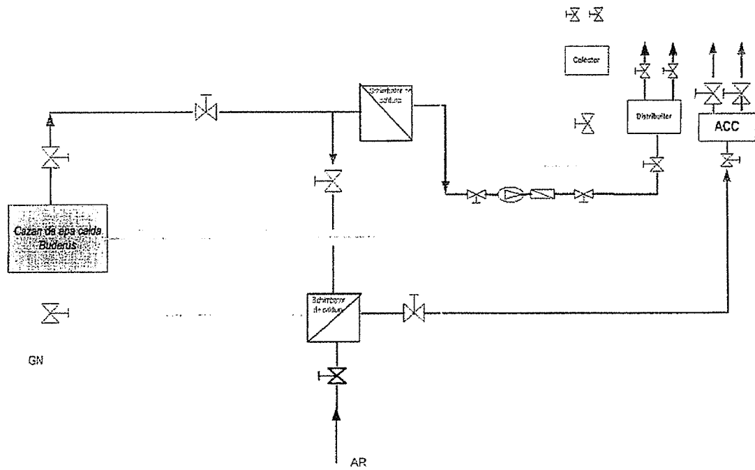
Schema termomecanică simplificată CT BISTRITA
