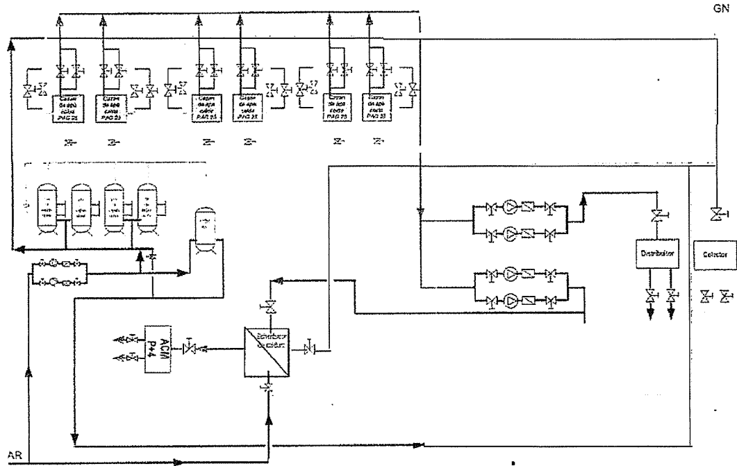
Schema termomecanica simplificata CT 3 Miorita
