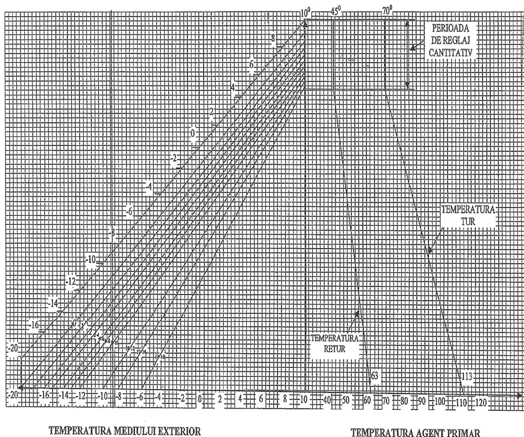
DIAGRAMA DE REGLAJ A LIVRĂRII AGENTULUI TERMIC PRIMAR
