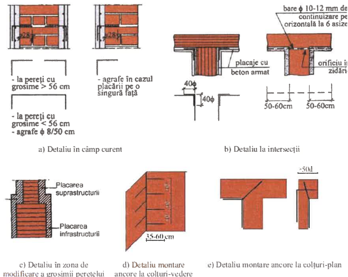
Fig.1 Exemple de camasuire a peretilor de zidarie utilizate in Romania
