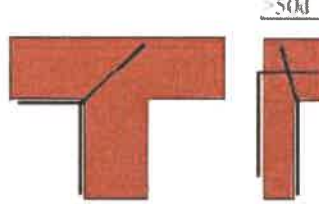
e) Detaliu montare ancore la colțuri-plan
