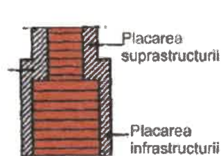
c) Detaliu în zona de modificare a grosimii peretelui
