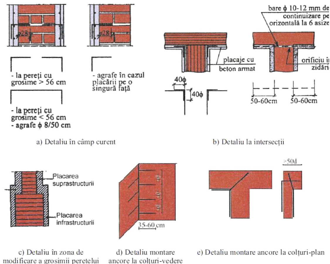
Fig.1 Exemple de camasuire a peretilor de zidarie utilizate in Romania
