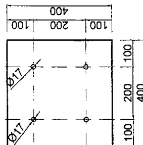
④ P4 PLACA INGRUPATA 400X400X10
