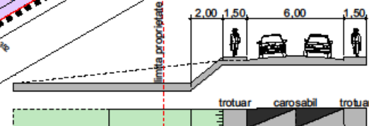
Profil transversal 1 strada COSTACHE NEGRUZI cat. a III-a sc. 1:200
