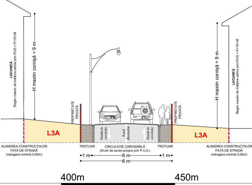
DRUM DE ACCES PROPUȘ - PROFIL STRADAL 8,00 m scara 1:200
