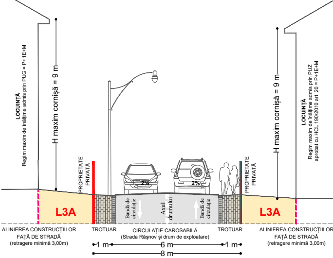
STR. RÂȘNOV ȘI DRUM DE EXPLOATARE - PROFIL STRADAL 8,00 m scara 1:200
