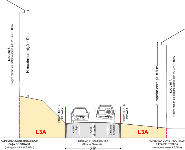
STRADA ZĂRNEȘTI - PROFIL STRADAL 6,00 m scara 1:200
