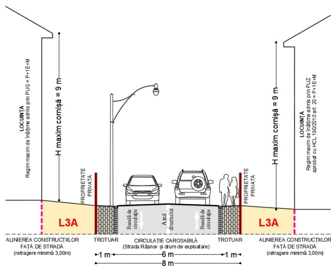
STR. RĂȘNOV ȘI DRUM DE EXPLOATARE - PROFIL STRADAL 8,00 m
