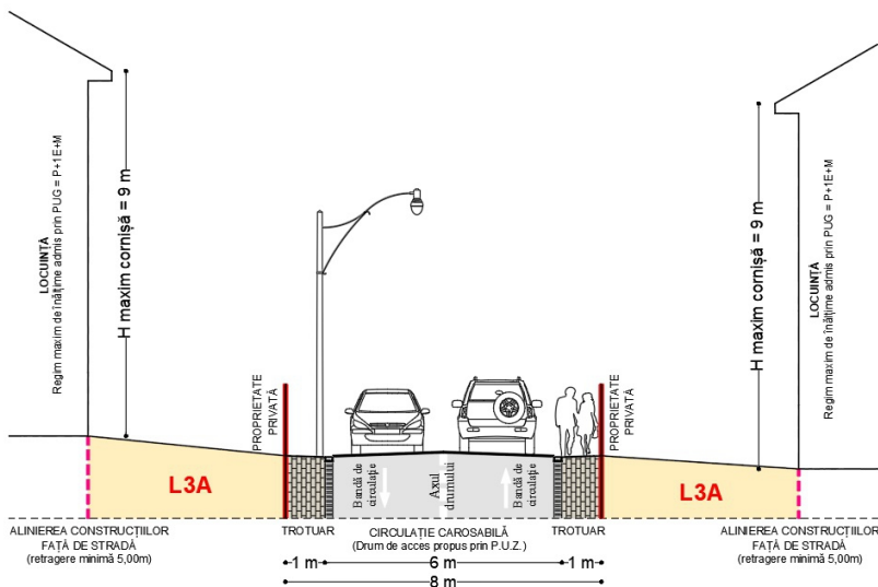
DRUM DE ACCES PROPUȘ - PROFIL STRADAL 8,00 m
