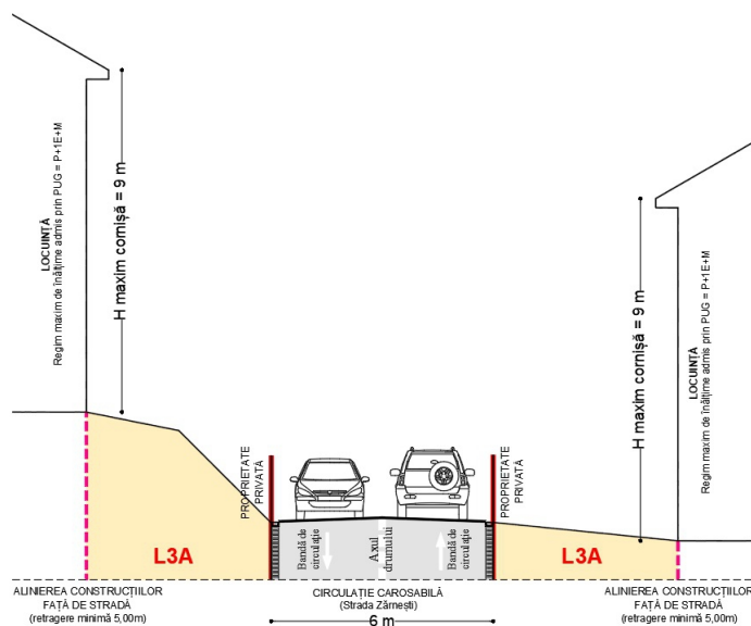
STRADA ZĂRNEȘTI - PROFIL STRADAL 6,00 m
