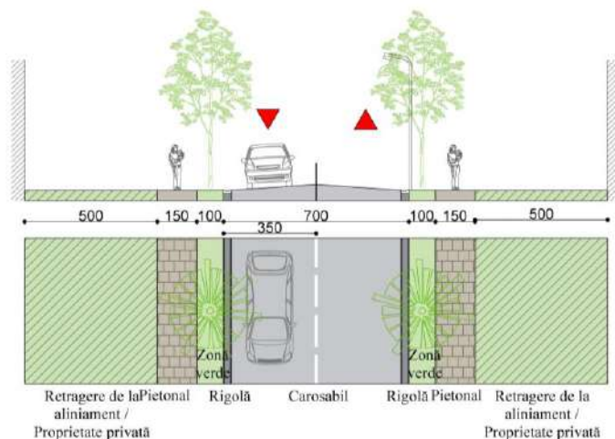
Secțiune A-A'
