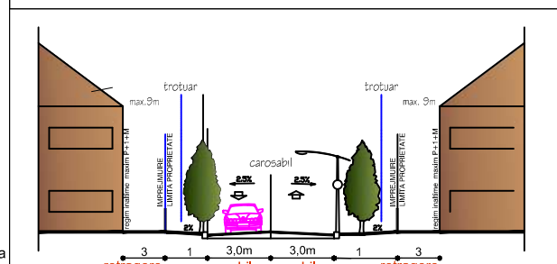
SECTIONE S - S SCARA 1 : 200
